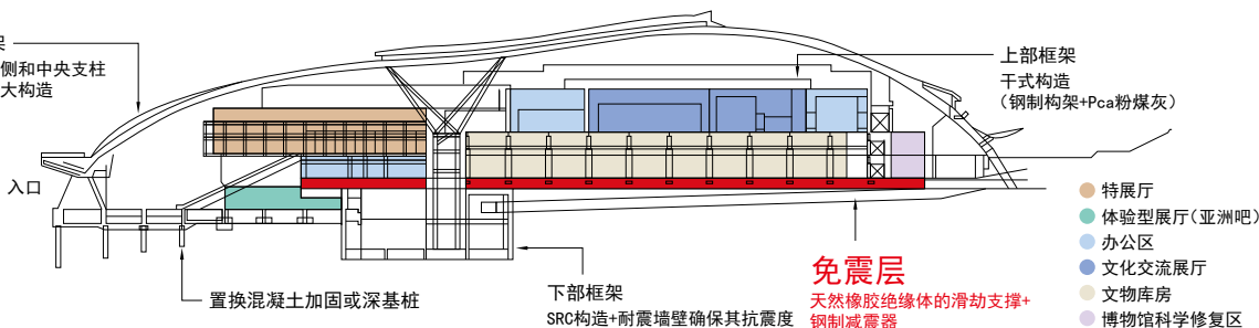
层压橡胶隔离器 (147个)
