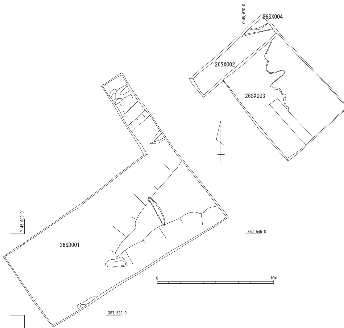
図 18. 遺構配置図 (1/200)
