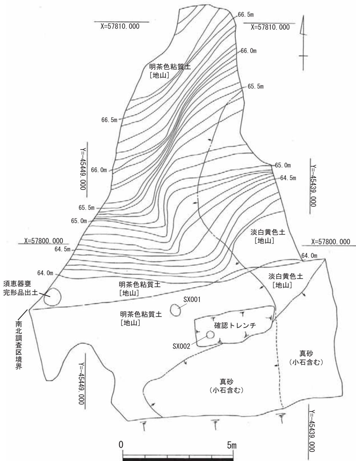
図 33. 遺構配置図 (1/100)
