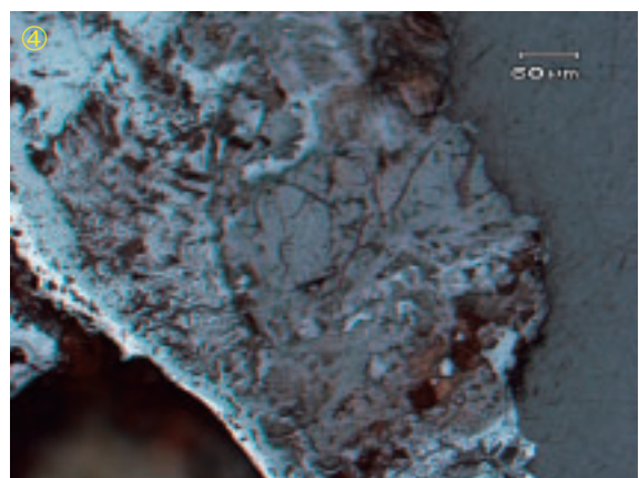
Photo.1 炉壁（含鉄）の顕微鏡組織
