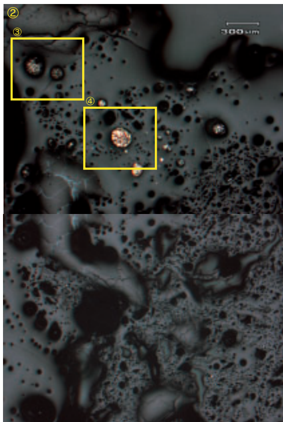
Photo.2 炉壁の顕微鏡組織
