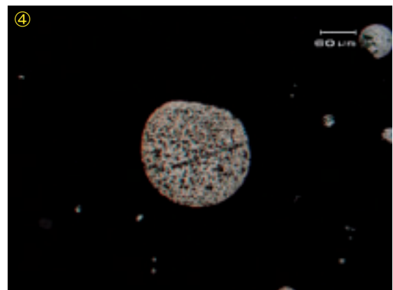
Photo.2 炉壁の顕微鏡組織
