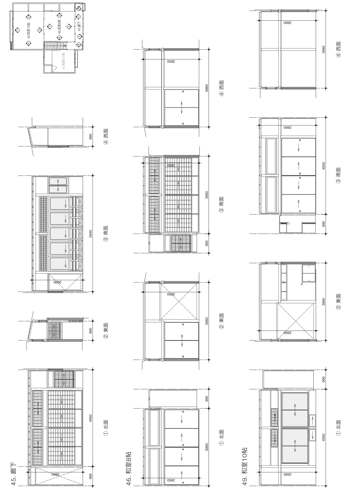
3・53 移築前展開図6 1:100
