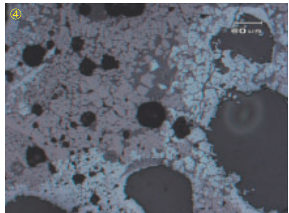
Photo.4 通風管の顕微鏡組織
