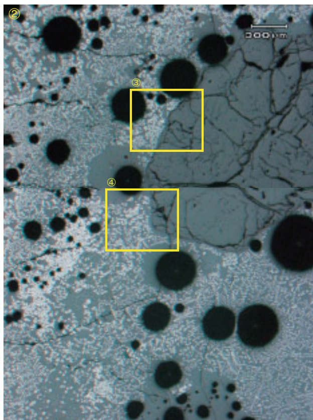
Photo.13 炉壁の顕微鏡組織
