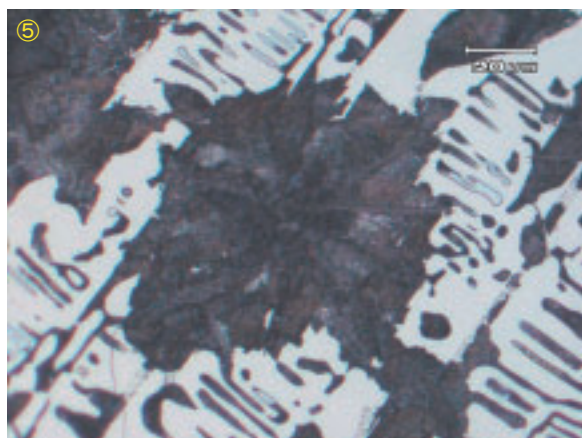
Photo.10 鉄塊系遺物の顕微鏡組織
