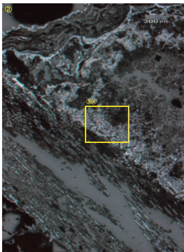
Photo.5 再結合滓の顕微鏡組織
