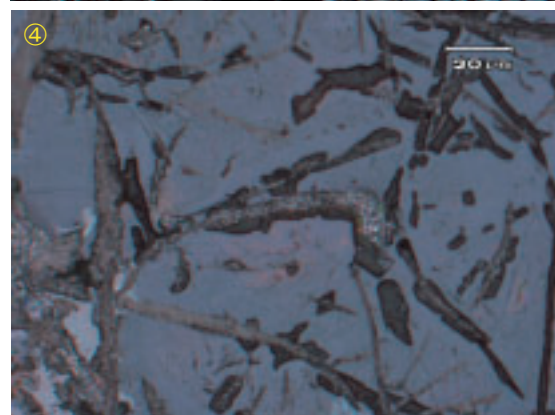
Photo.5 再結合滓の顕微鏡組織
