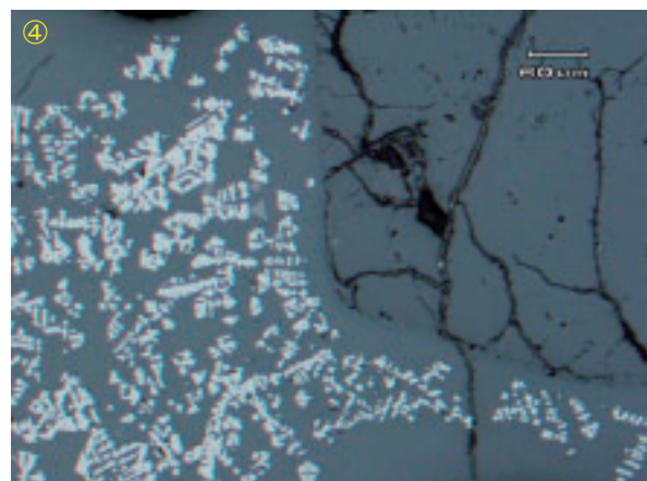
Photo.13 炉壁の顕微鏡組織
