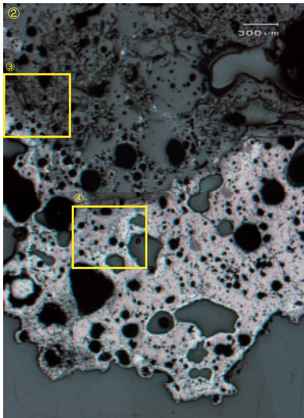
Photo.4 通風管の顕微鏡組織
