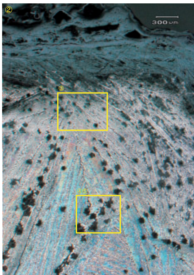
Photo.10 鉄塊系遺物の顕微鏡組織
