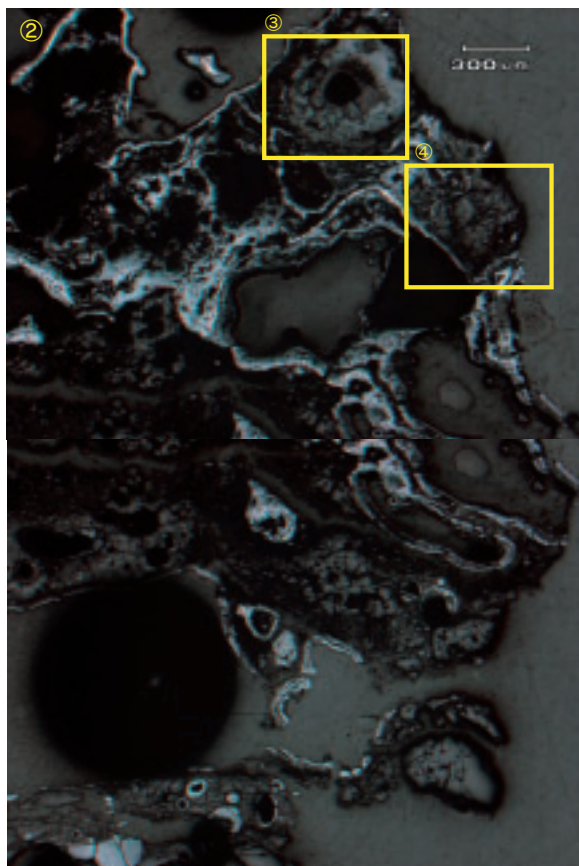
Photo.1 炉壁（含鉄）の顕微鏡組織
