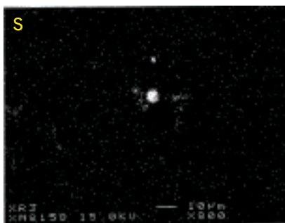
Photo.8 炉壁（含鉄）の顕微鏡組織・EPMA調査結果
