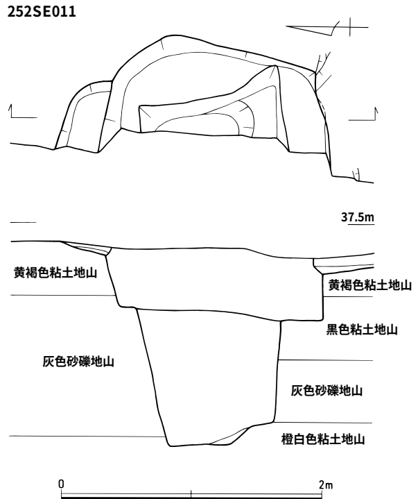
第9図 252SE011実測図（1/40）
