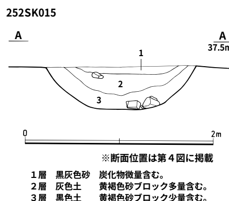
第11図 252SK015土層断面実測図 (1/40)
