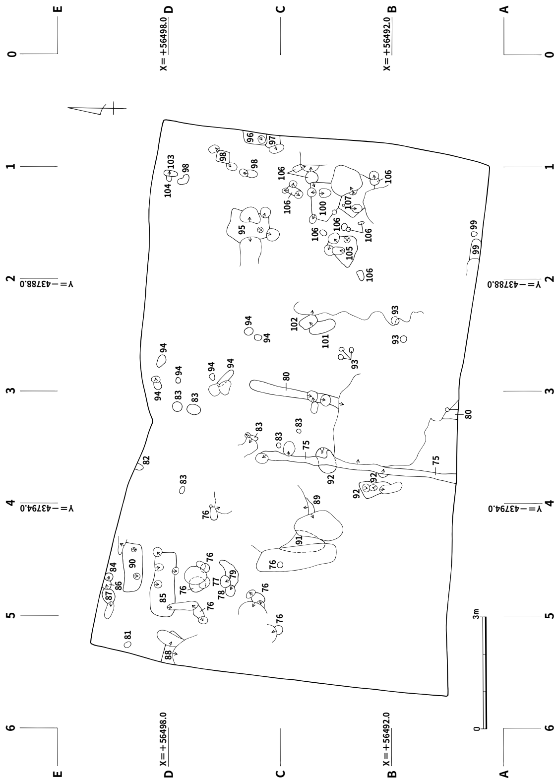
第22図 大宰府条坊跡第252次調査第II面遺構配置図 (1/100)
