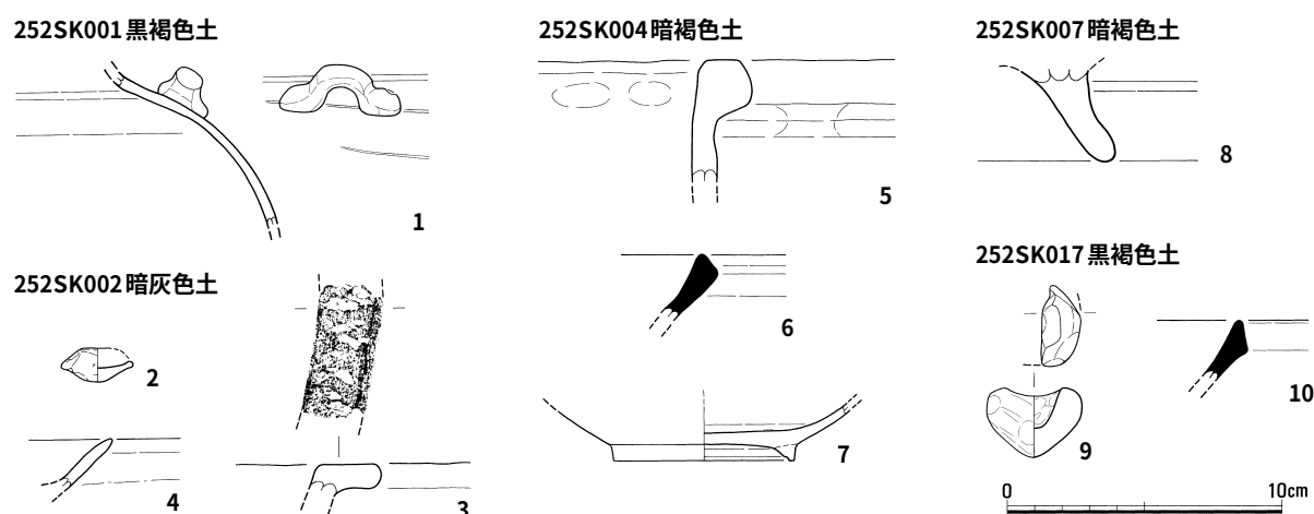
第14図 252SK001・002・004・007・017出土遺物実測図 (1/3)
