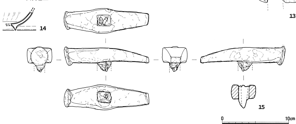
第35図 233SE035遺物実測図 (1/3)
