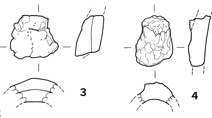
第30図 233SD018・040遺物実測図（1/3）
