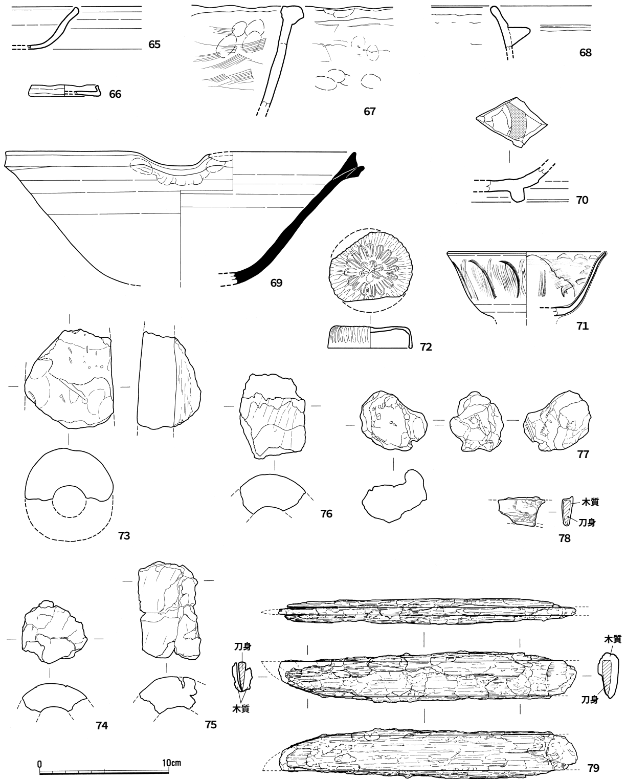
第27図 233SD005遺物実測図4 (1/3)
