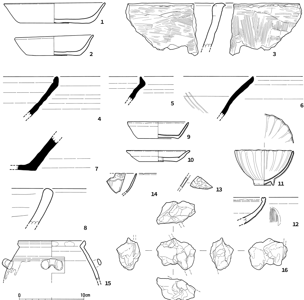
第46図 233SX036遺物実測図1 (1/3)
