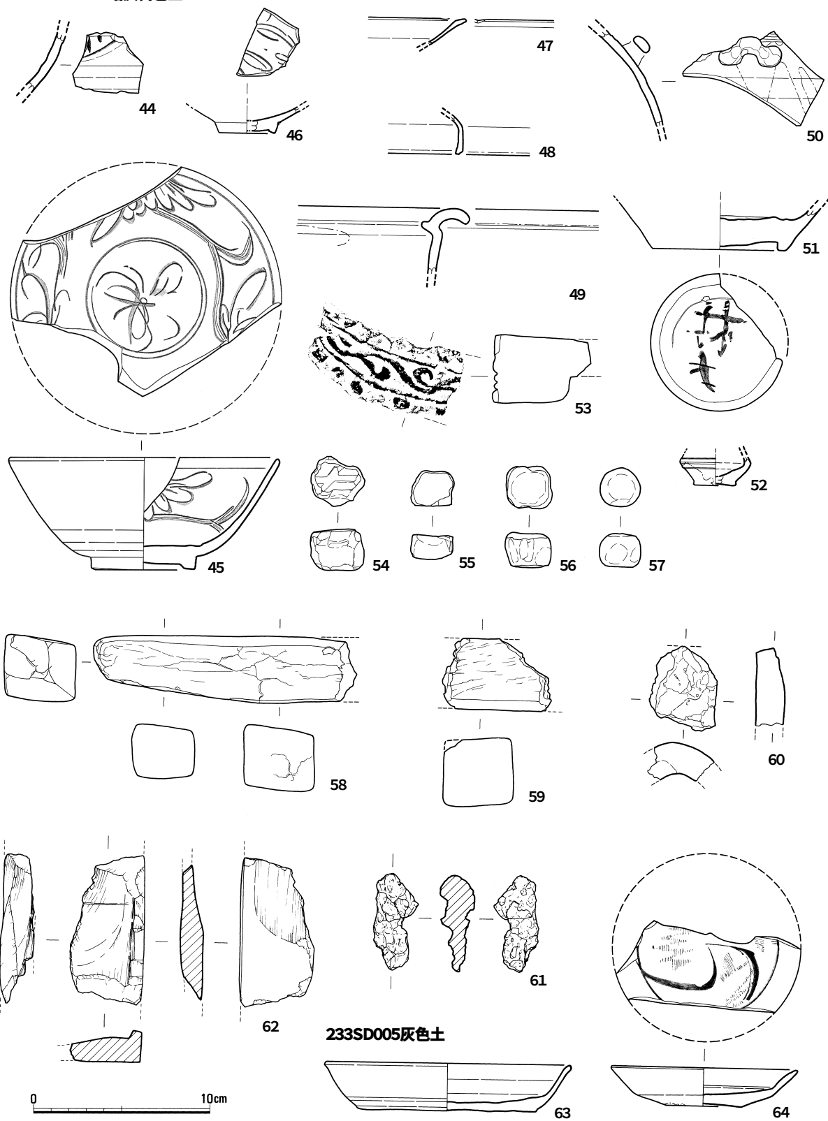
第26图 233SD005遺物実測図3 (1/3)
