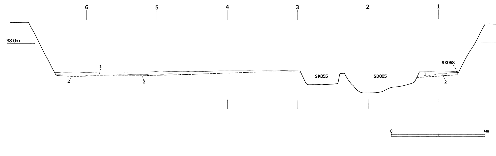
第8図 1・2号トレンチ土層断面図 (1/80)
