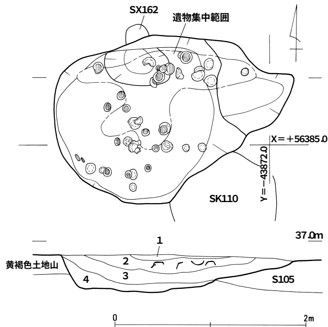
第23図 233SK095実測図 (1/40)
