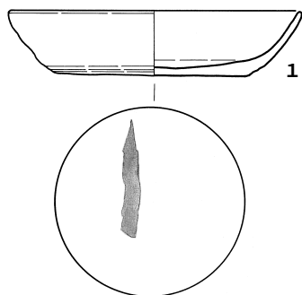
第32図 233SD077・105・115・120遺物実測図 (1/2・1/3)
