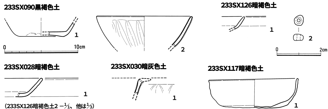
第48図 233SX028・030・090・117・126遺物実測図 (1/1・1/3)
