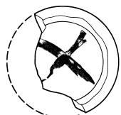
第25图 233SD005遺物実測図2 (1/3)
