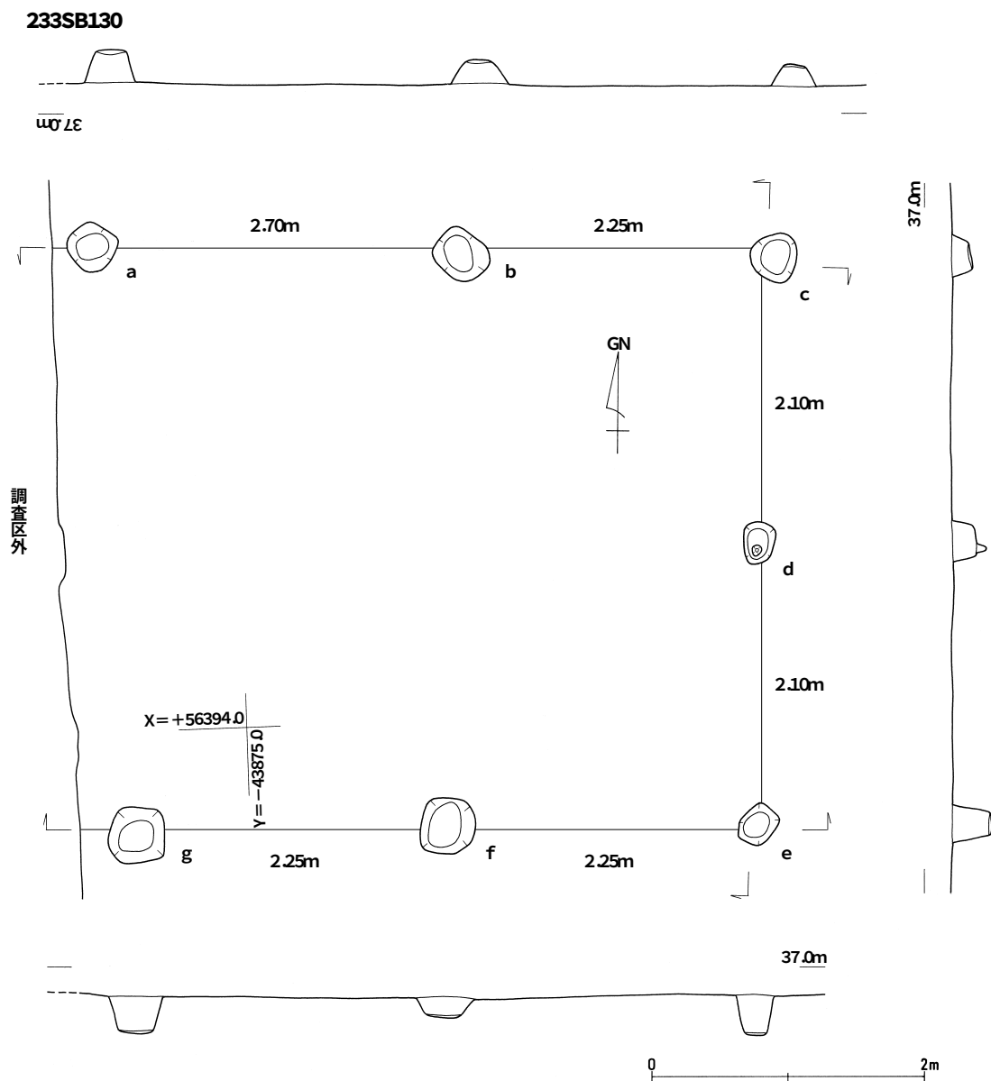
第18図 233SB130実測図 (1/50)
