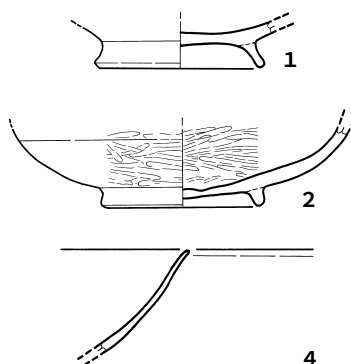
第33図 233SE010・011・015遺物実測図（1/3）
