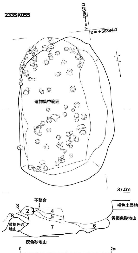
第22図 233SK055実測図 (1/40)
