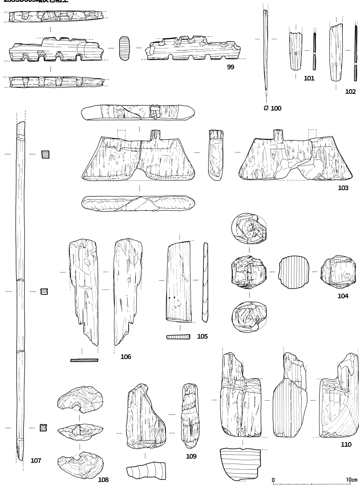
第29图 233SD005遺物実測図6 (1/3)
