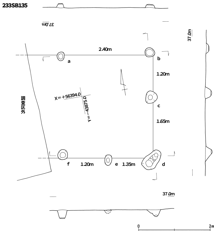
第19図 233SB135実測図 (1/50)
