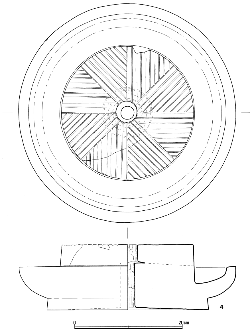
第37図 233SE050遺物実測図 (1/3・1/4)
