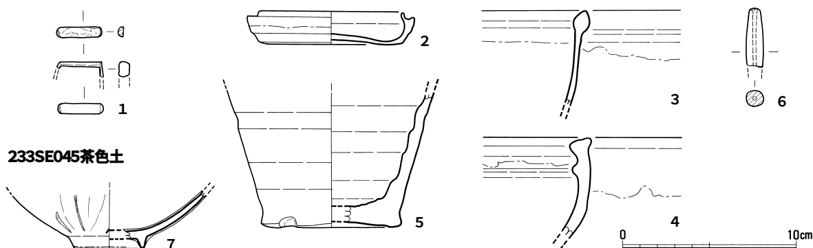
第36図 233SE045遺物実測図 (1/3)
