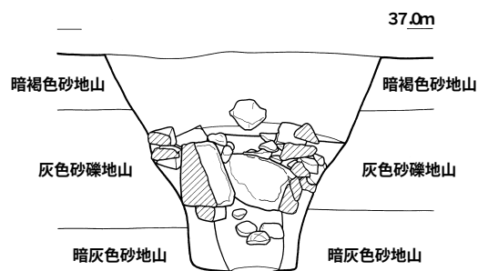
第12図 233SE003・010・011実測図 (1/50)
