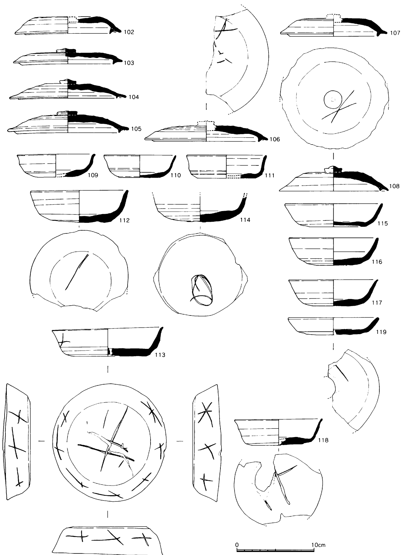
fig.18 神ノ前遺跡第2次調査 SX005黒灰褐色土出土遺物実測図 その2 (1/3)
