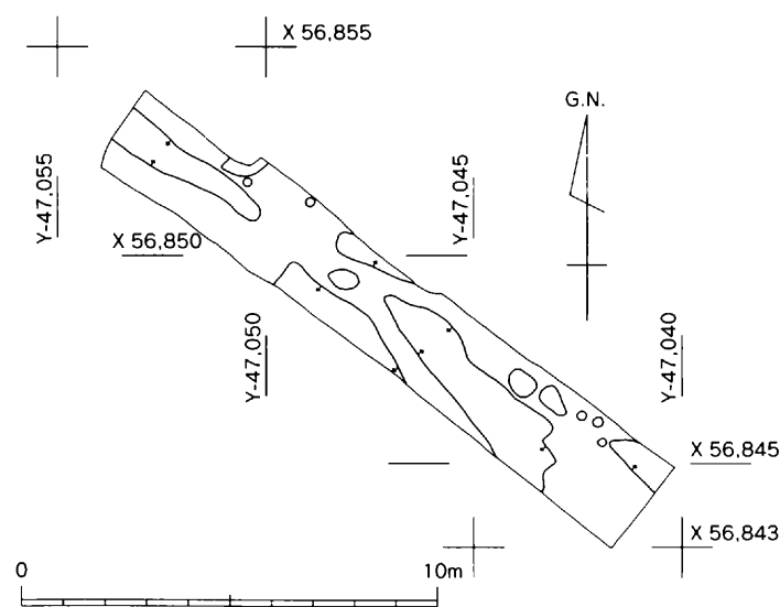
fig.23 島本遺跡第1次調査 遺構配置図 (1/200)
