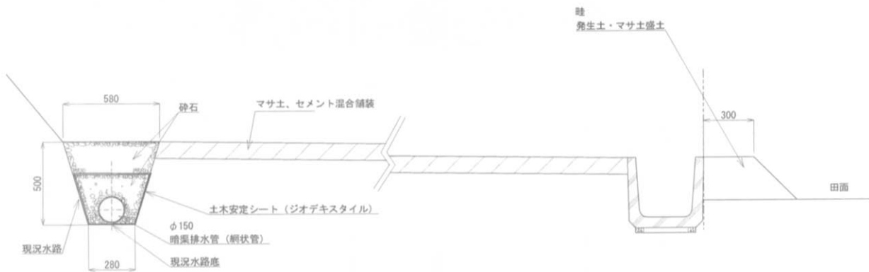
Fig.37 管理通路標準図
