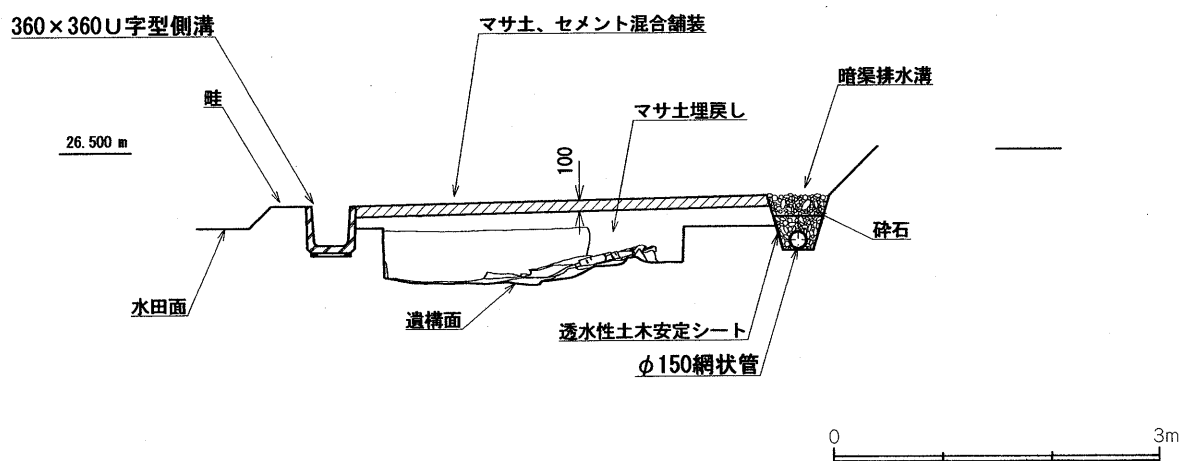
Fig.40 第31次調査2号瓦窯付近整備図
