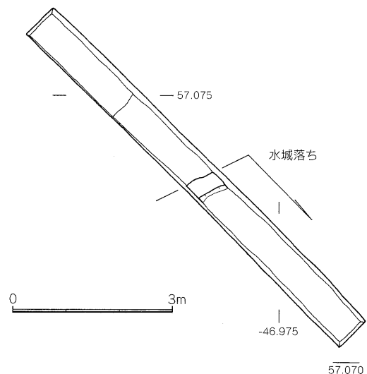
Fig.28 トレンチ3遺構実測図（1/100）
