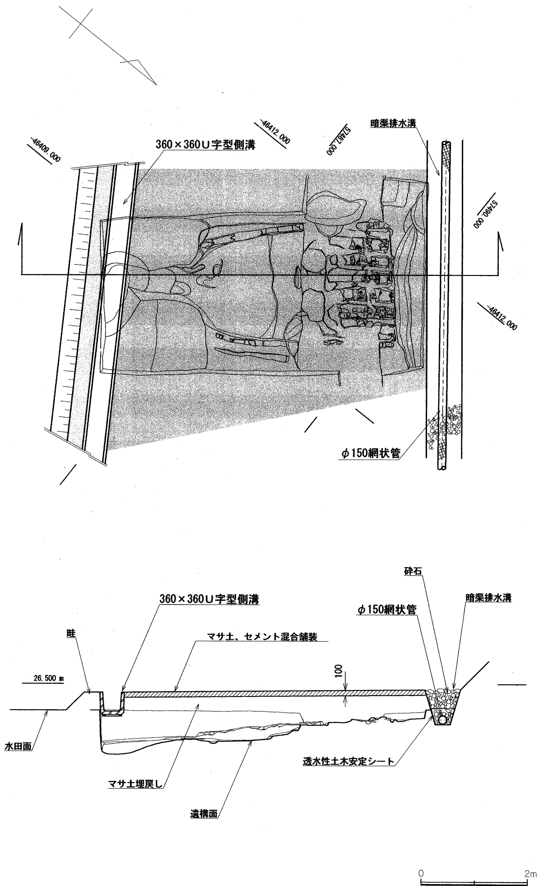
Fig.39 第31次調査1号瓦窯付近整備図
