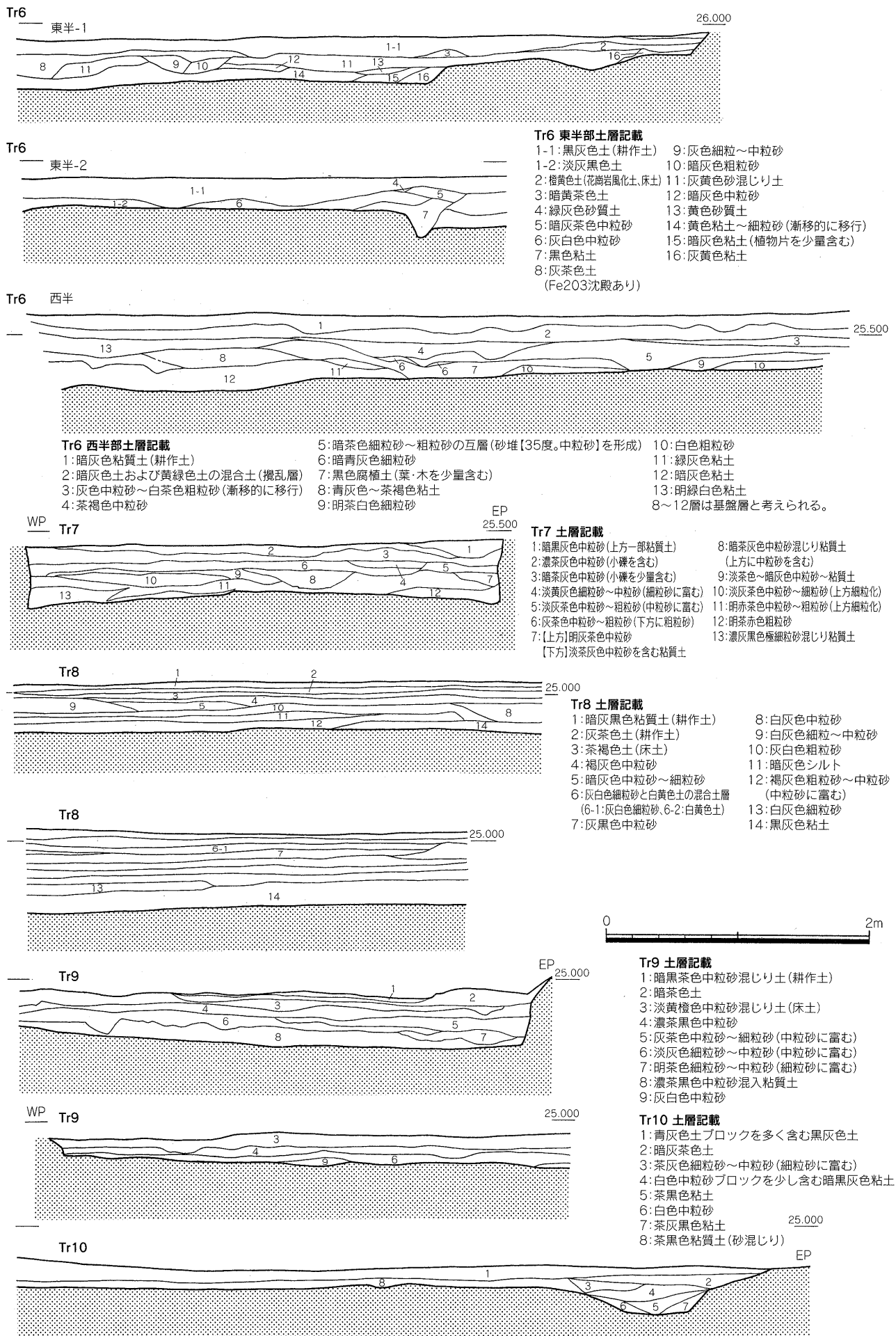
Fig.11 第31次調査Tr6~T10土層実測図 (1/40)
