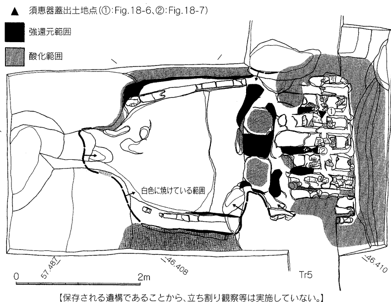
Fig.13 31SX001 (1号瓦窯) 遺構配置図 (1/60)
