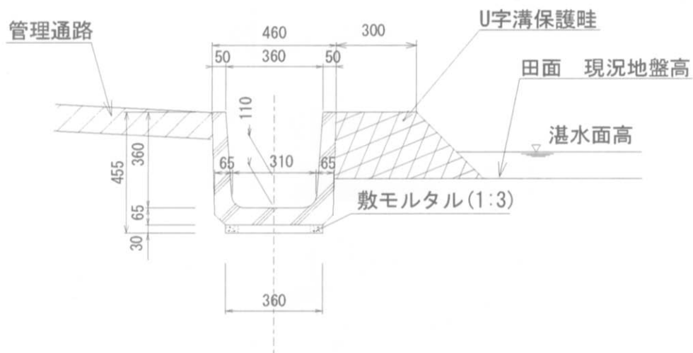
Fig.36 U字型側溝布設標準図
