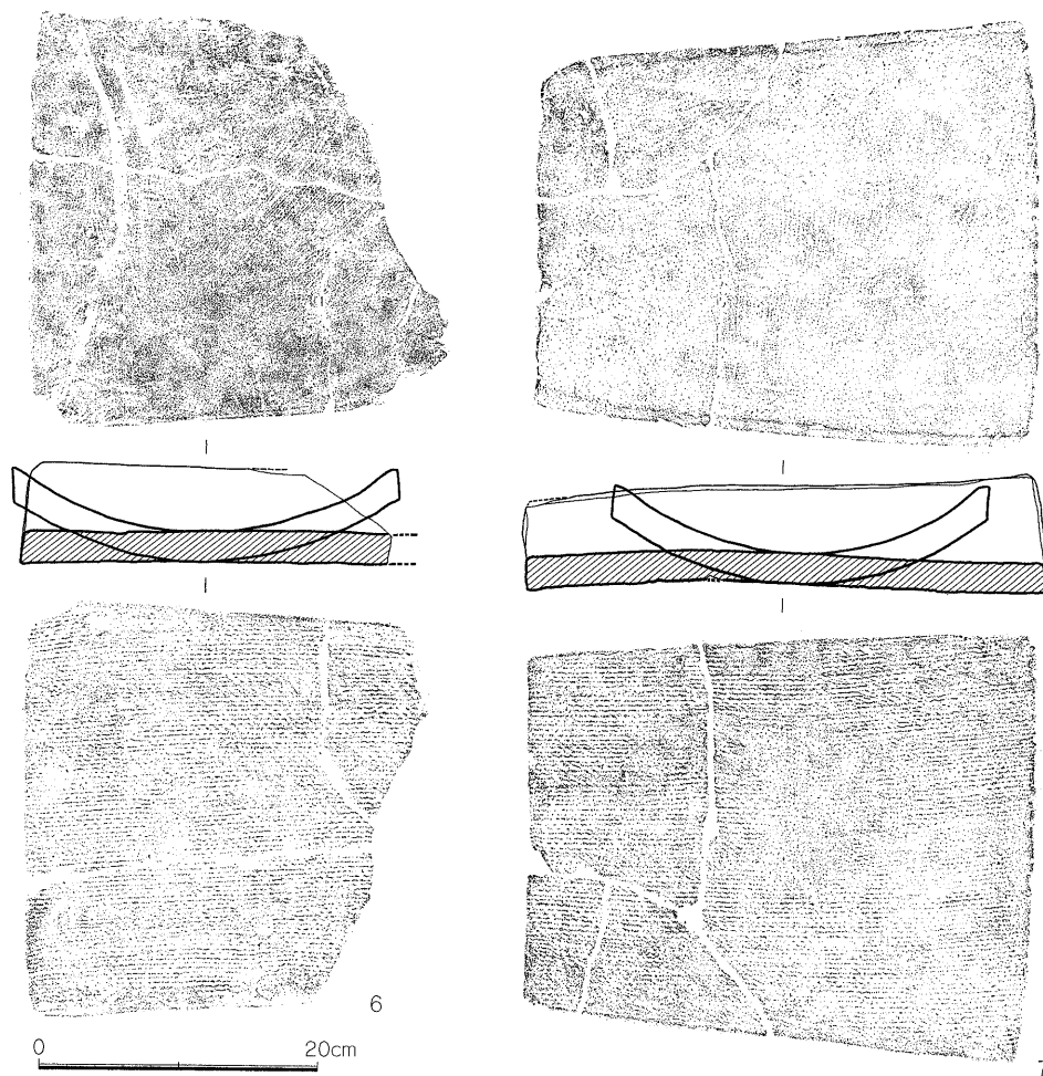
Fig.21 31SX002 (2号瓦窯) 出土遺物実測図3 (1/6)
