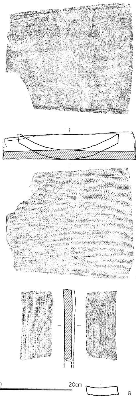
Fig.22 31SX002 (2号瓦窯) 出土遺物実測図4 (1/6)
