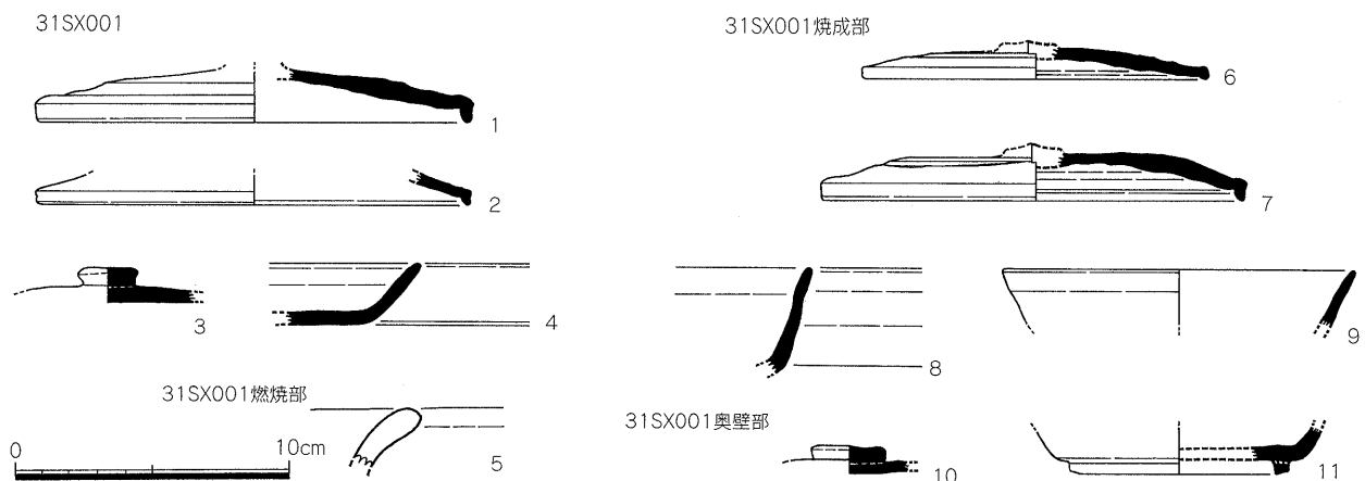
Fig.18 31SX001（1号瓦窯）出土遺物実測図（1/3）
