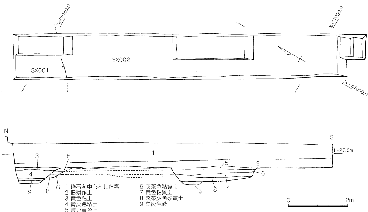
Fig.3 第28次調査全体図および東壁土層図 (1/40)
