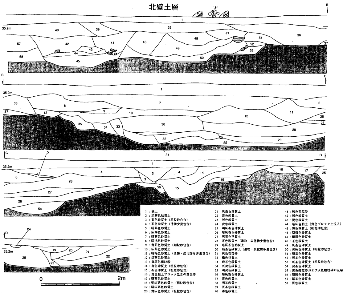
図3.基本土層実測図 (S=1/60)
