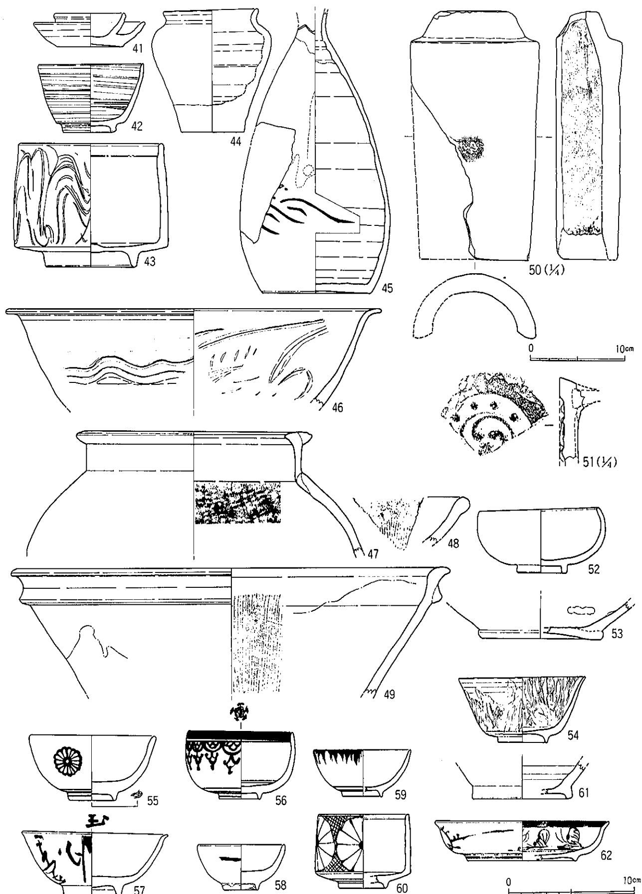
Fig.11 第1区出土遺物実測図2 (1/3・1/4)
