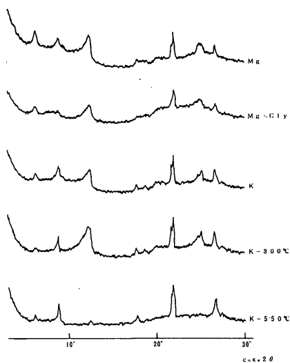
図1 池ノ口遺跡 黒灰色土X線回析チャート
