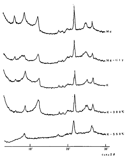
図2 池ノ口遺跡 灰褐色土X線回析チャート
