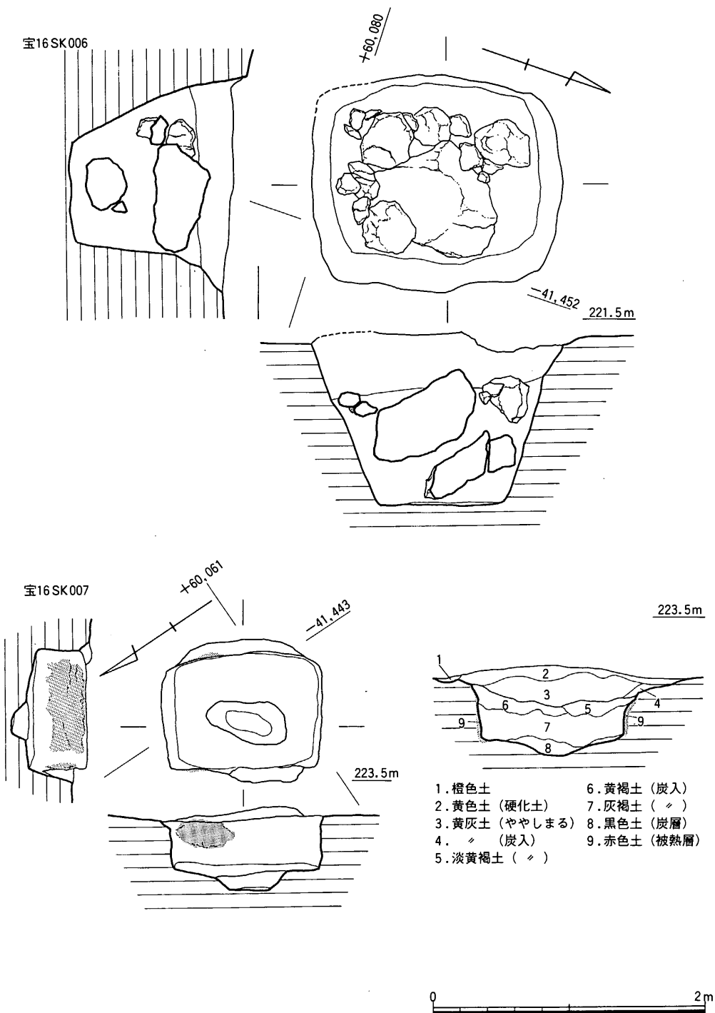
第19図 宝満16次B区遺構実測図2 (1/40)
