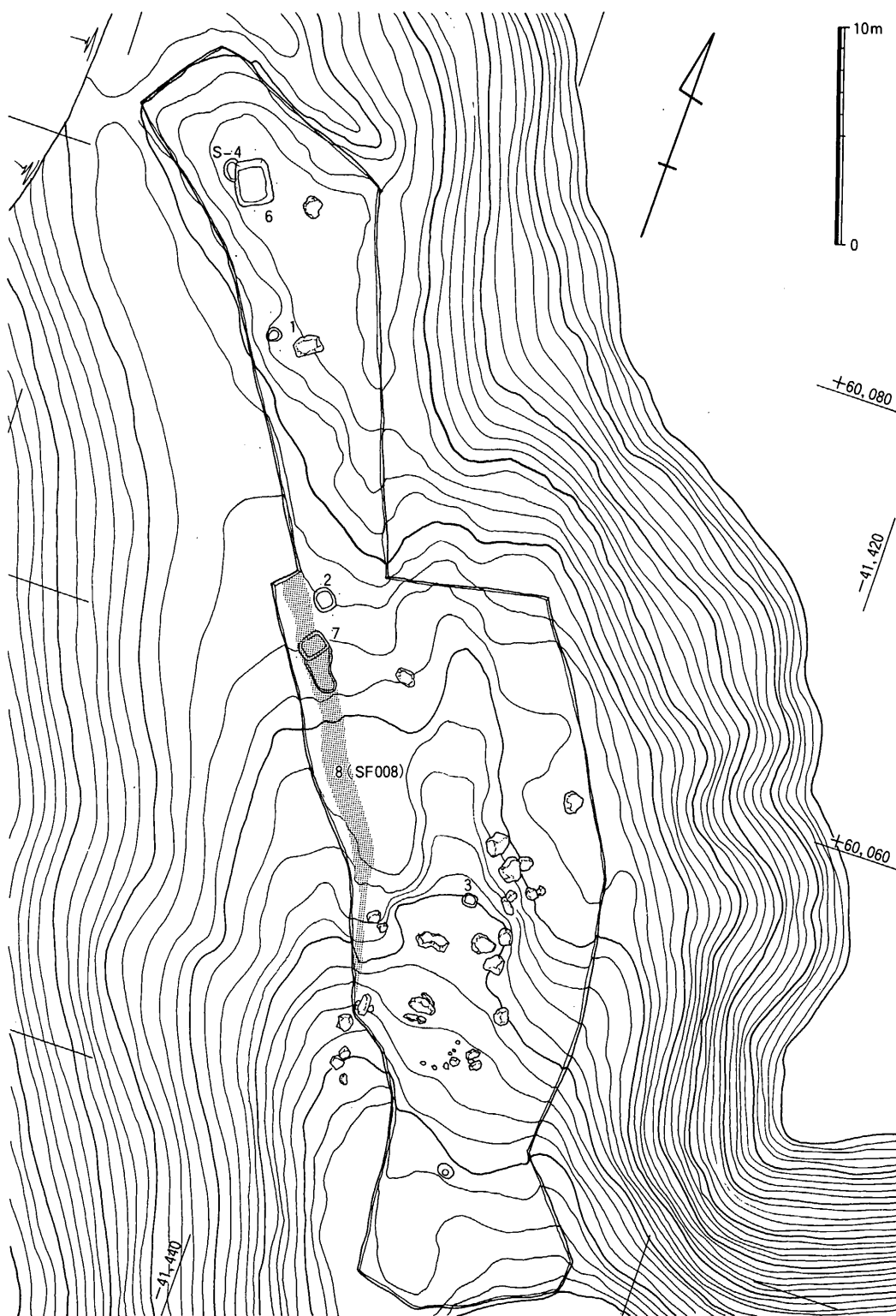
第17図 宝満16次調査区全体図2
