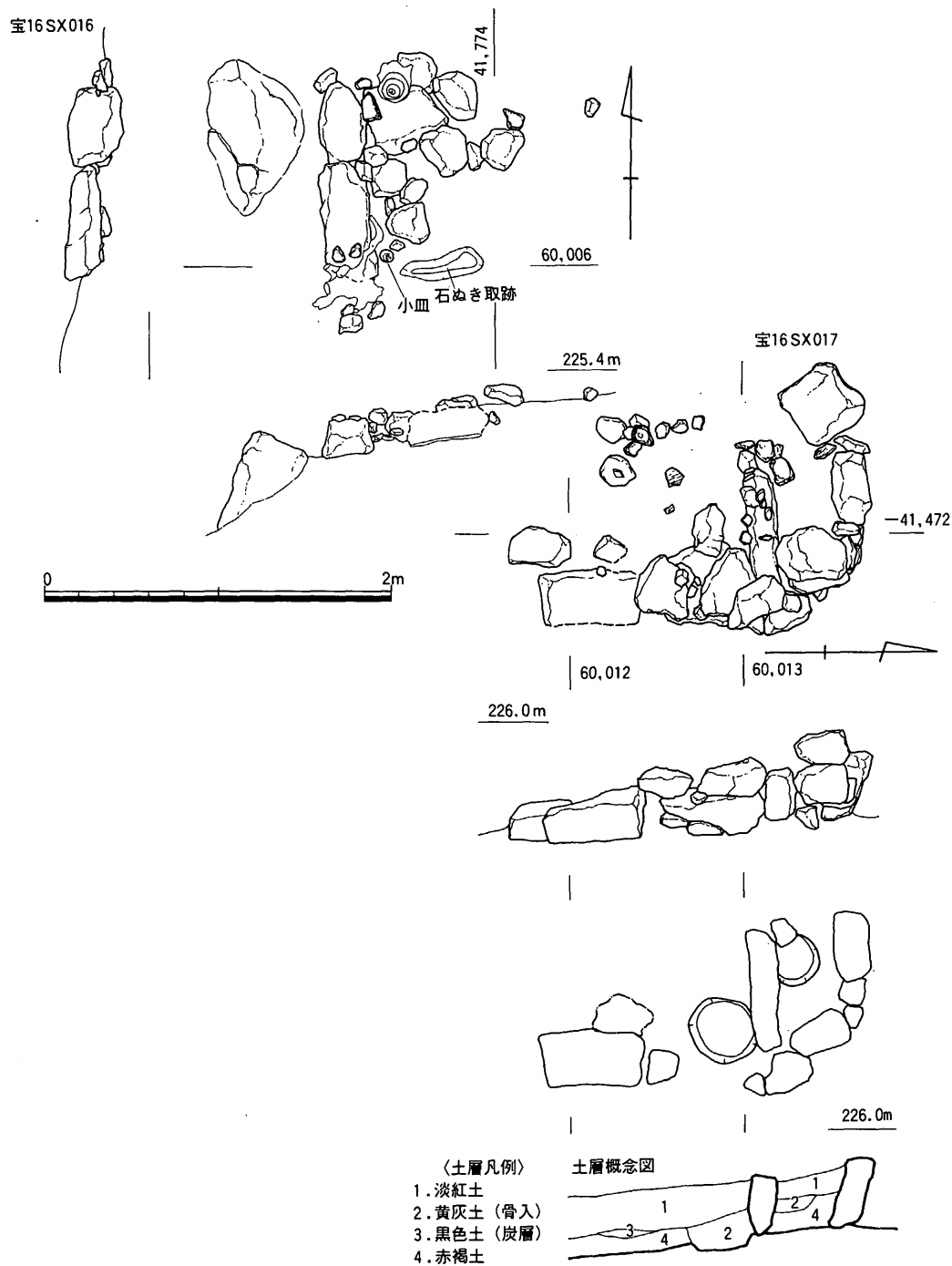
第14図 宝満16次A区遺構実測図4 (1/40)
