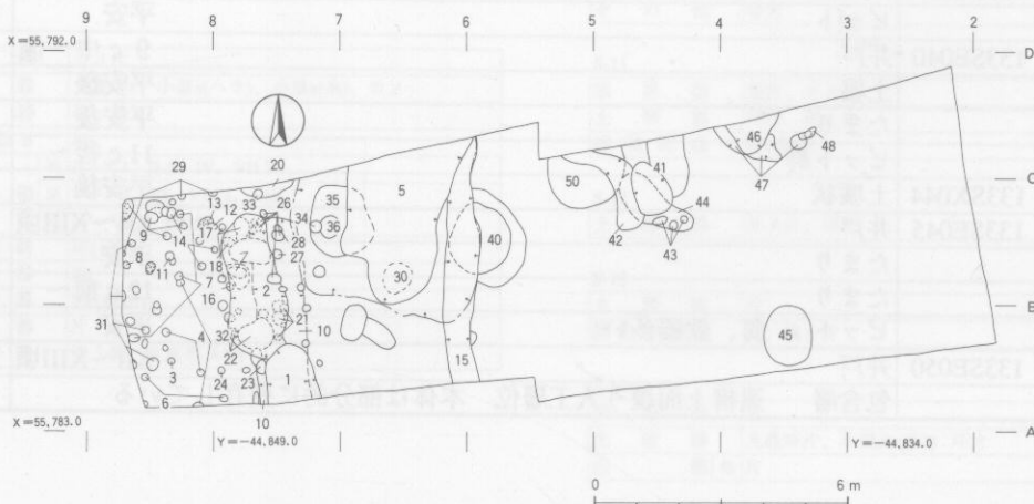
大宰府条坊跡 第133次調査 遺構配置図 (1/200)
