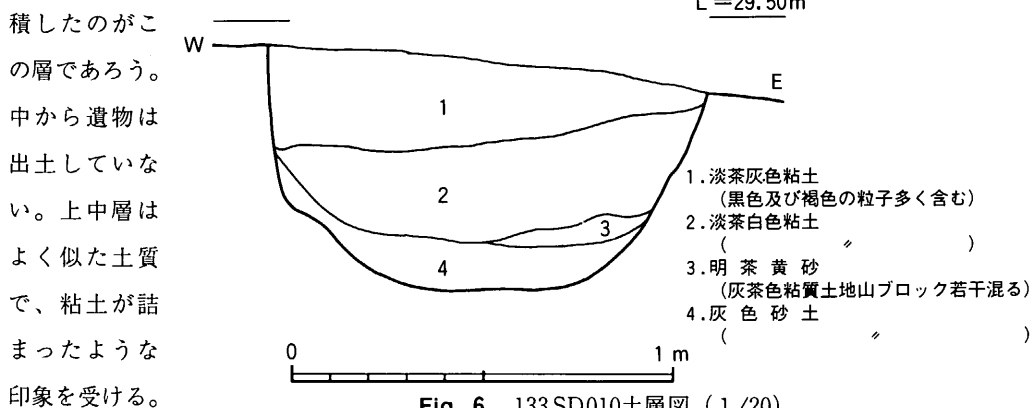
Fig. 6 133SD010土層図 (1/20)
