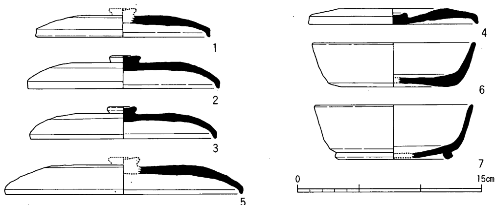
Fig.23 1号窯跡床面出土土器実測図
