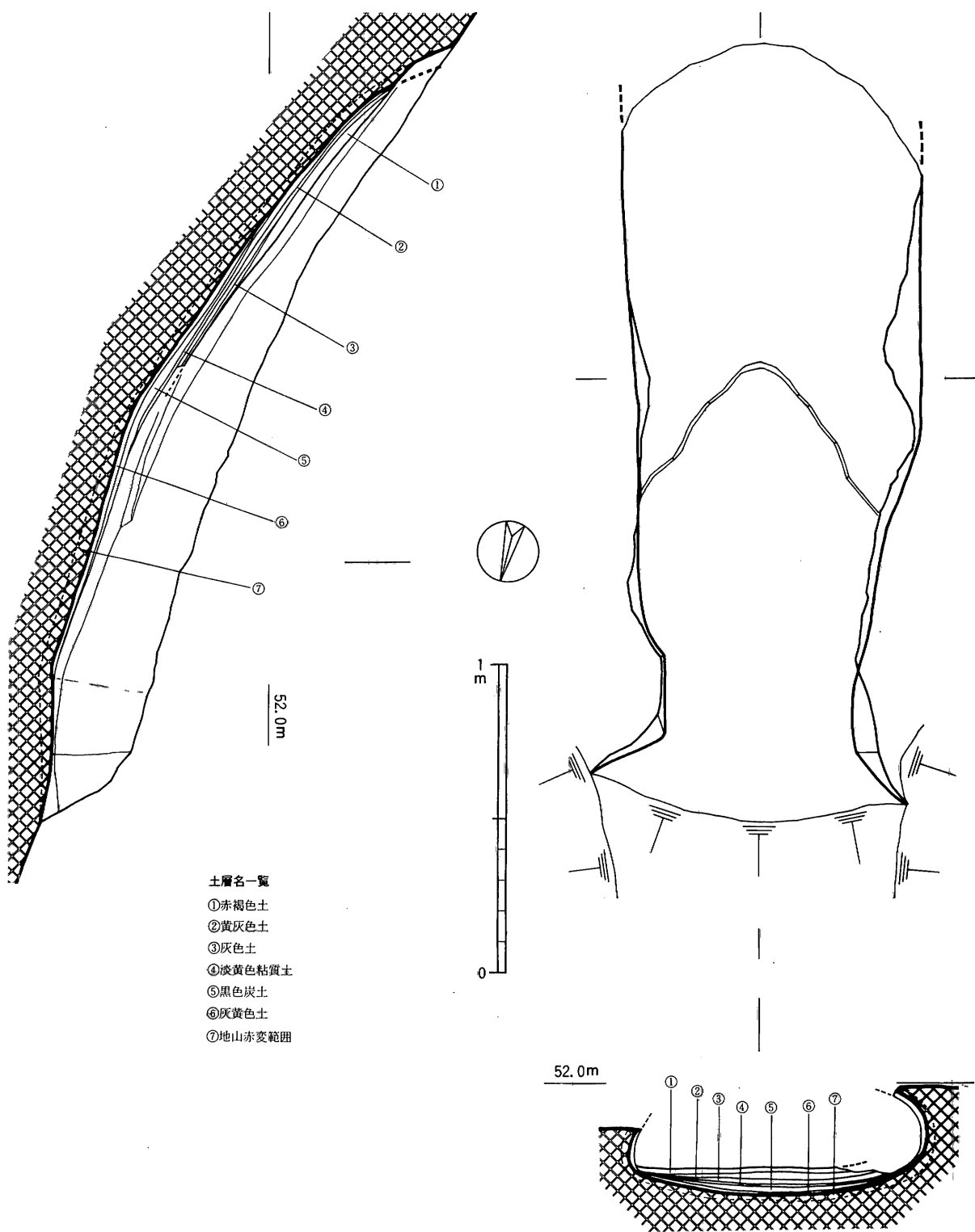
Fig.25 2号窯跡実測図
