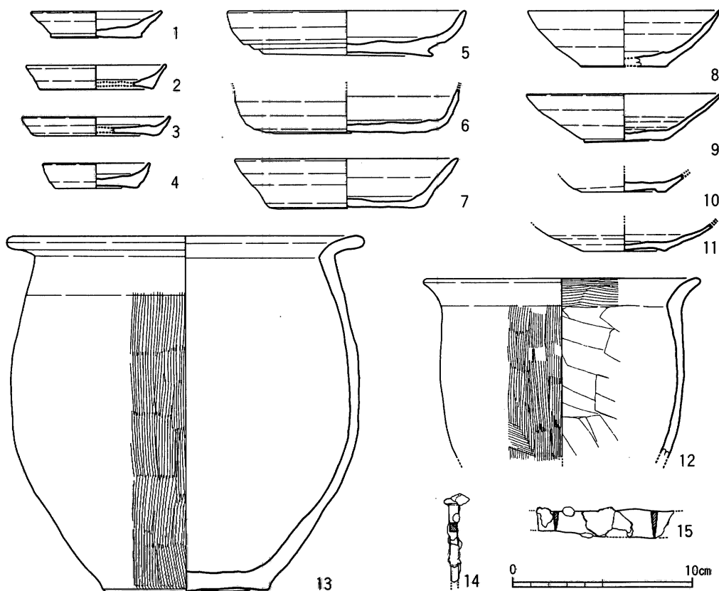
Fig.12 SX001出土遺物実測図
