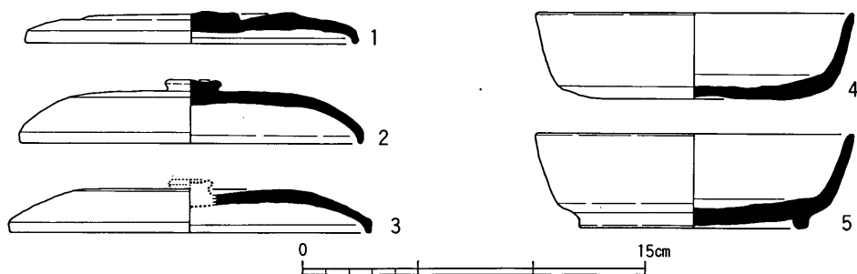
Fig.24 1号窯跡埋土中出土土器実測図
