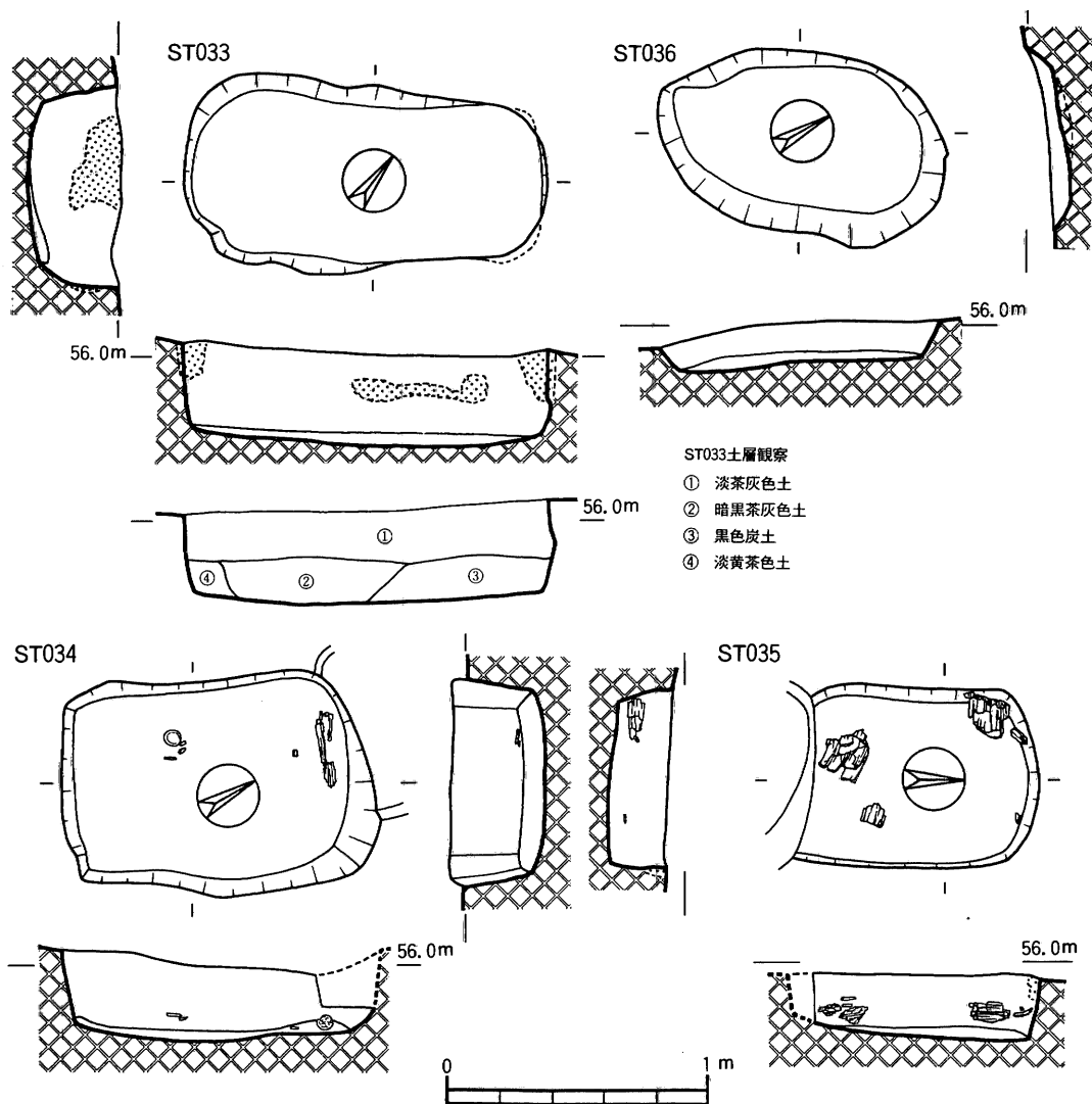
Fig.17 火葬施設実測図(2)
