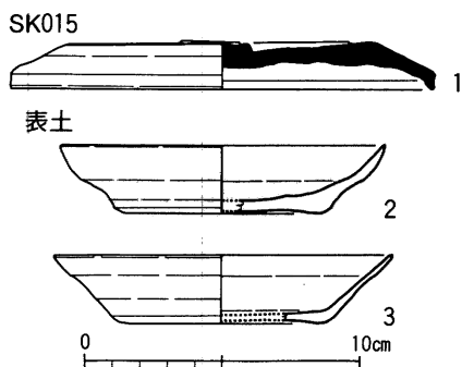
Fig.28 SK015・表土出土土器実測図
