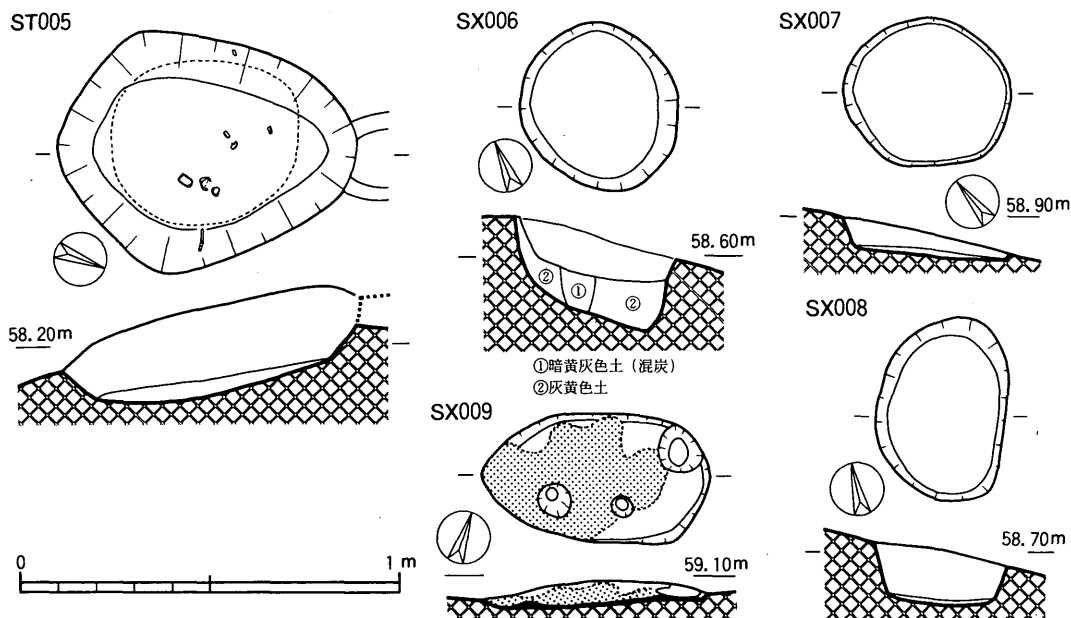
Fig. 5 西調査区検出遺構実測図
