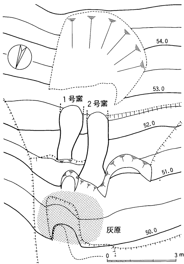
Fig.21 1・2号窯跡周辺地形測量図
