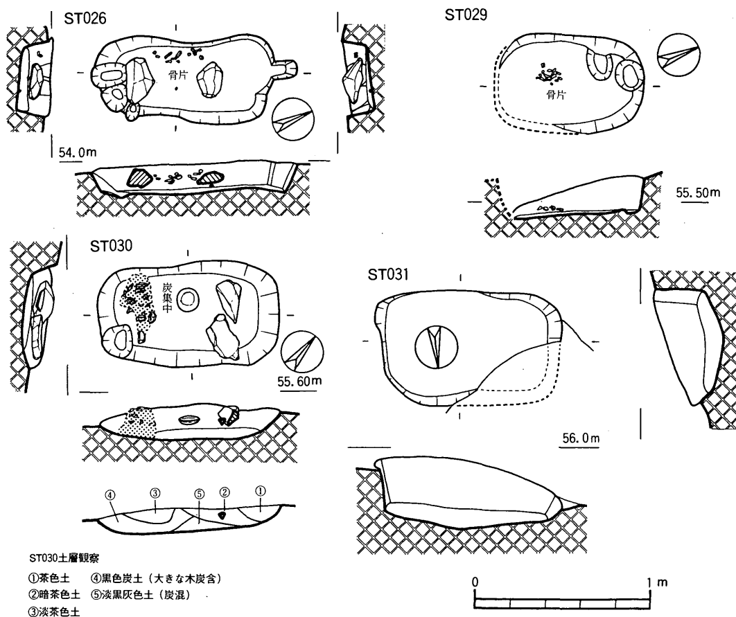
Fig.16 火葬施設実測図(1)
