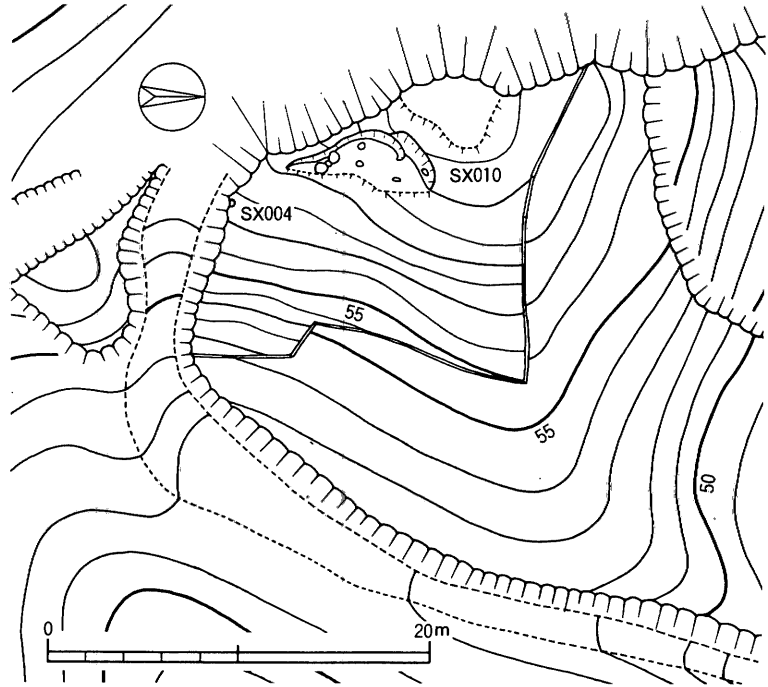
Fig. 3 西調査区地形測量図
