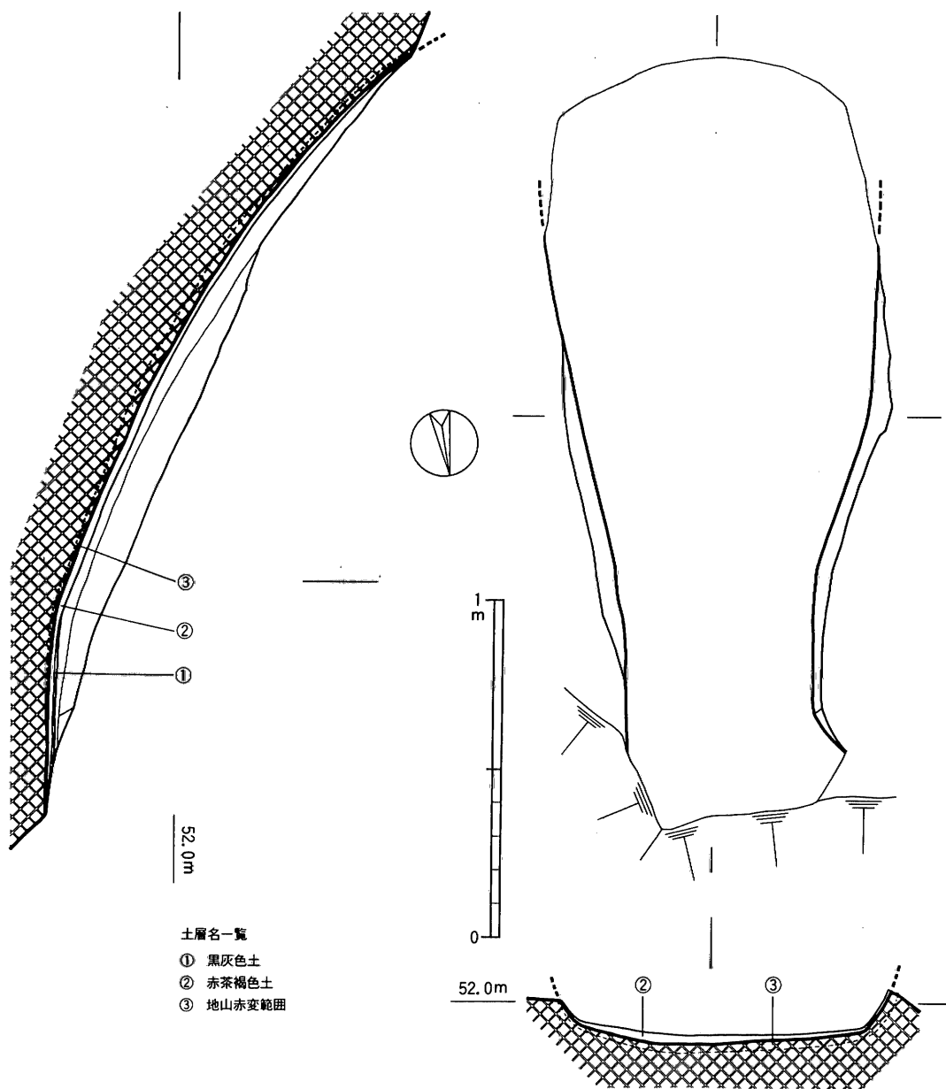
Fig.22 1号窯実測図
