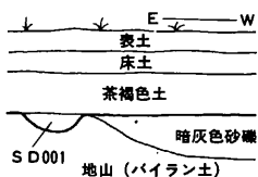
図4 土層模式図
