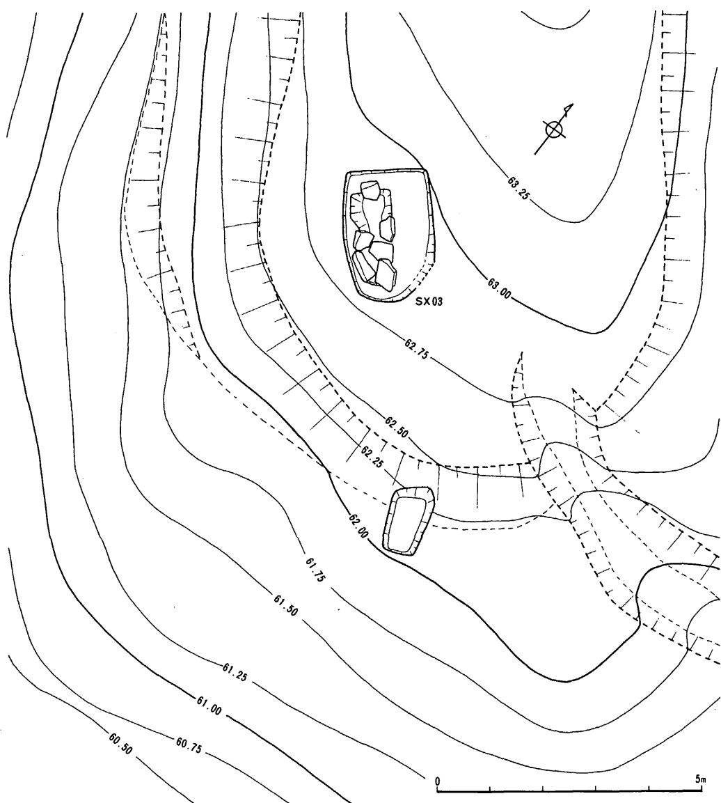
図12 SX03周辺地形図（地山コンタ）（1/100）
