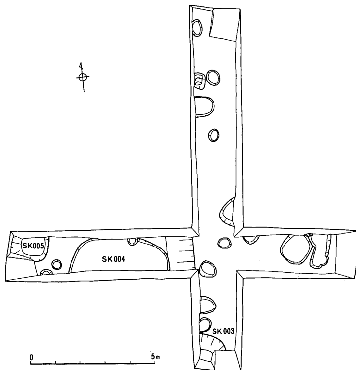
図6 第2次調査遺構配置図 (1/150)
