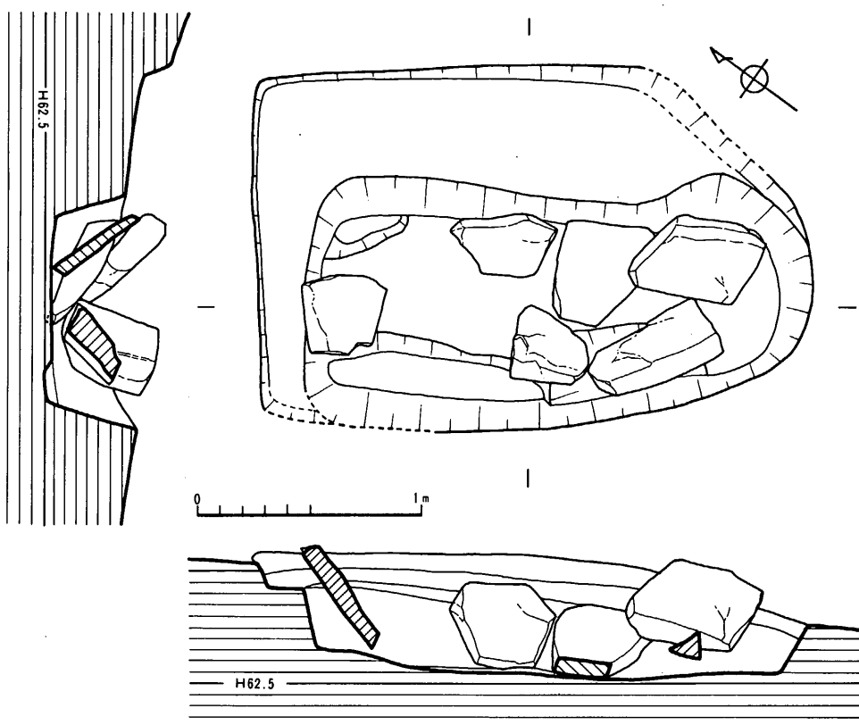
图13 SX03实测图 (1/30)
