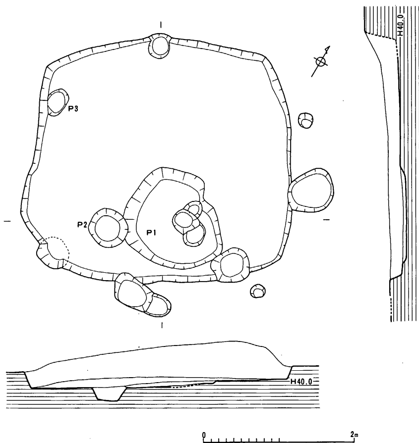
図11 SB01実測図 (1/50)
