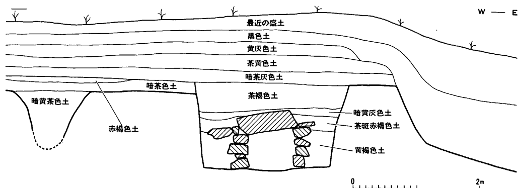
図21 SX01土層図 (1/60)
