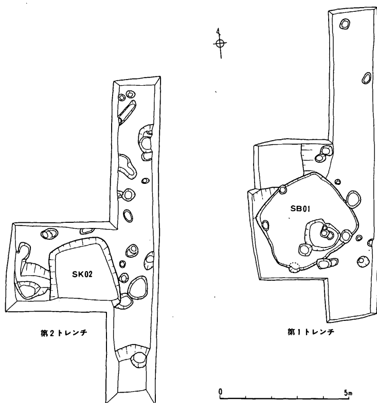
図10 第1次調査、第1・2トレンチ遺構配置図 (1/150)
