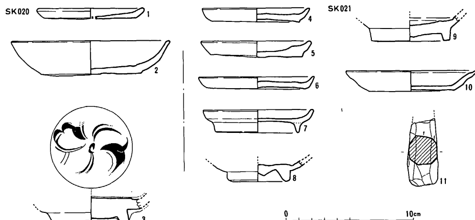
図18 SK020・021出土遺物 (1/3)
