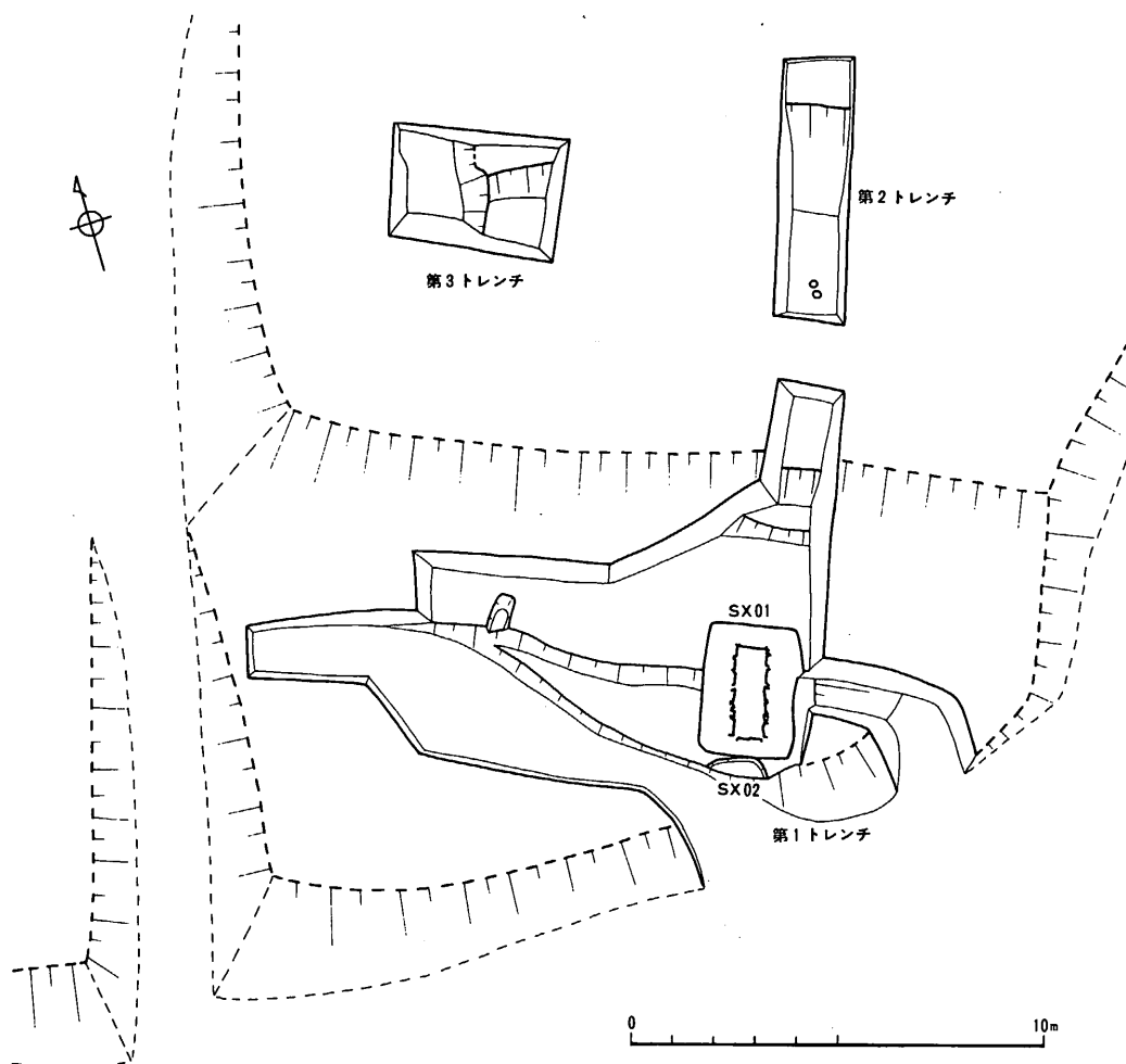
図20 遺構配置図 (1/200)
