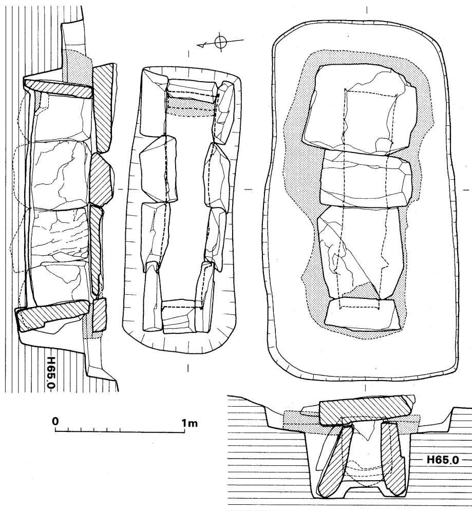
Fig. 8 2号墳主体 (1/30)
