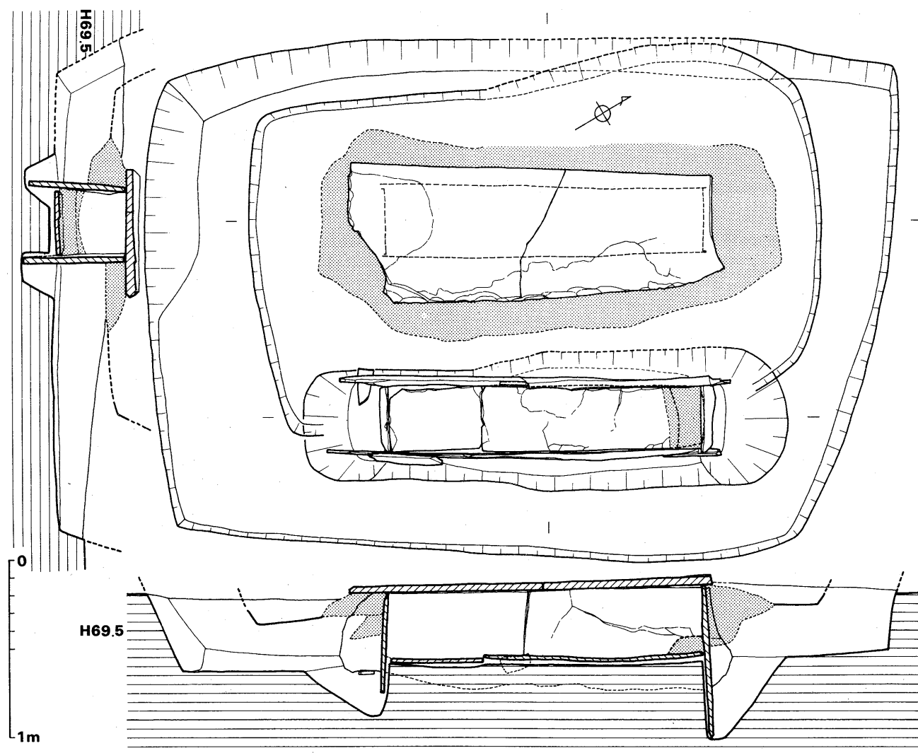
Fig. 14 6号墳主体 (1/30)
