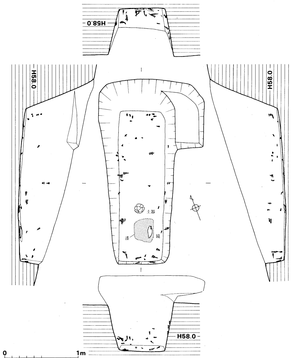
Fig.36 3 号 墓 (1/30)
