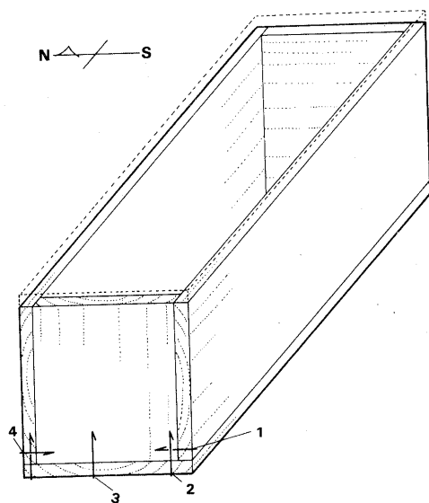
Fig.34 2号墓木棺推定図
