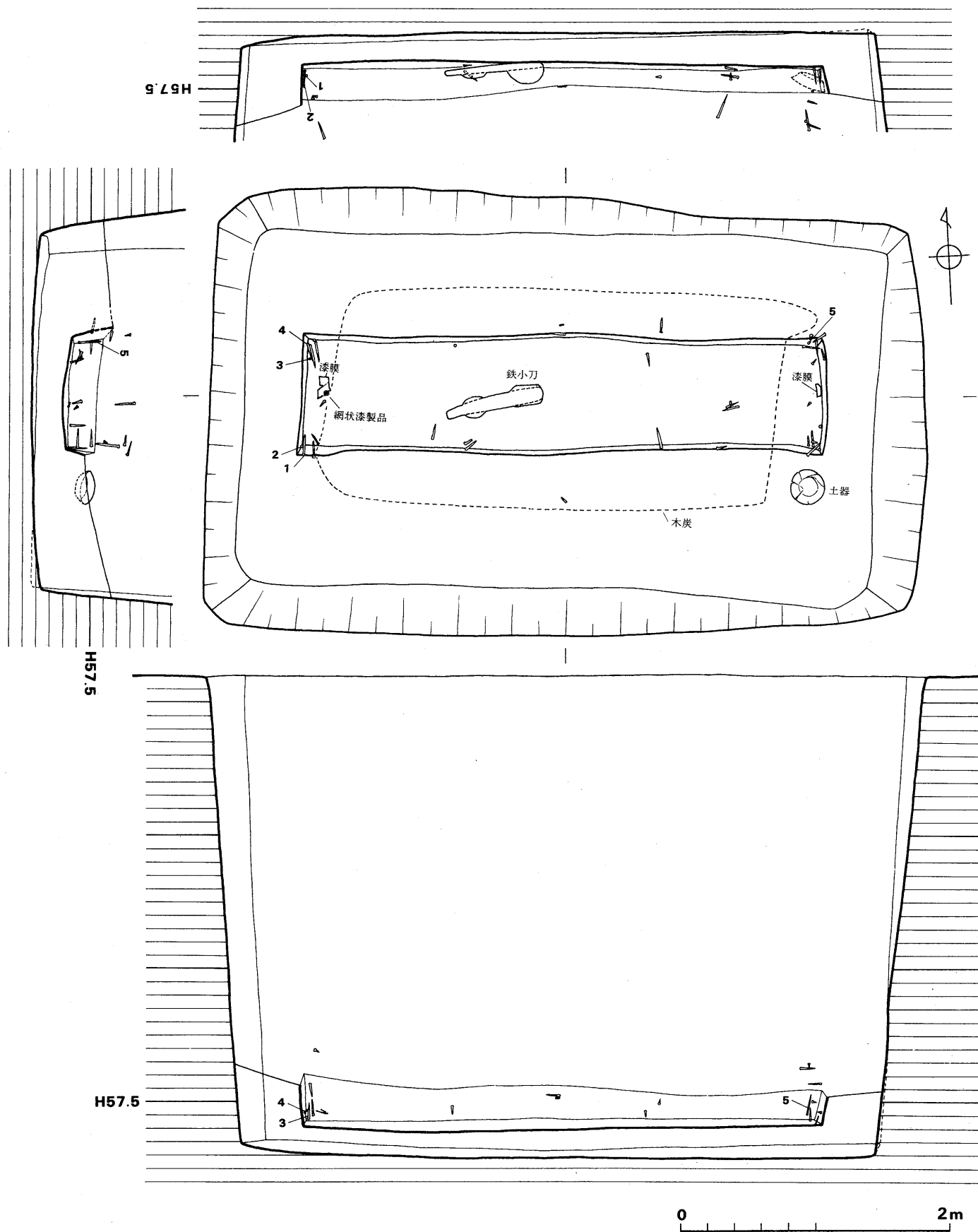
Fig.31 2 号 墓 (1/20)
