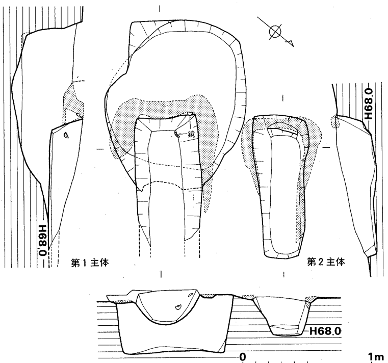
Fig.12 5号墳主体 (1/30)
