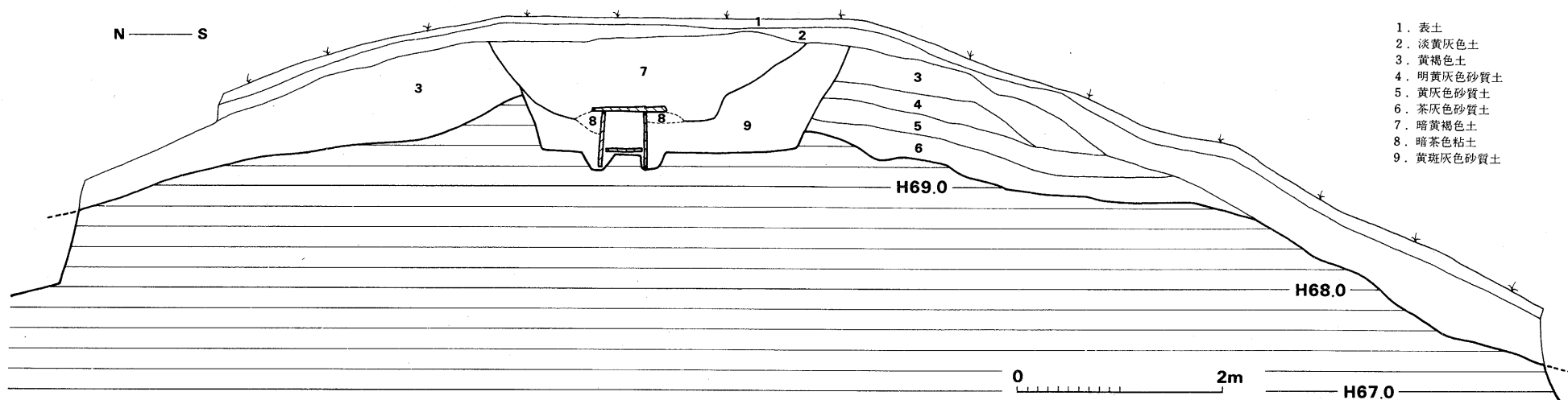
Fig. 13 6号墳土層図 (1/60)
