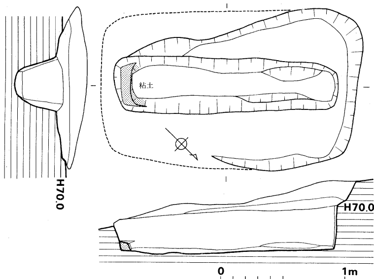
Fig.19 1号土壇墓 (1/30)
