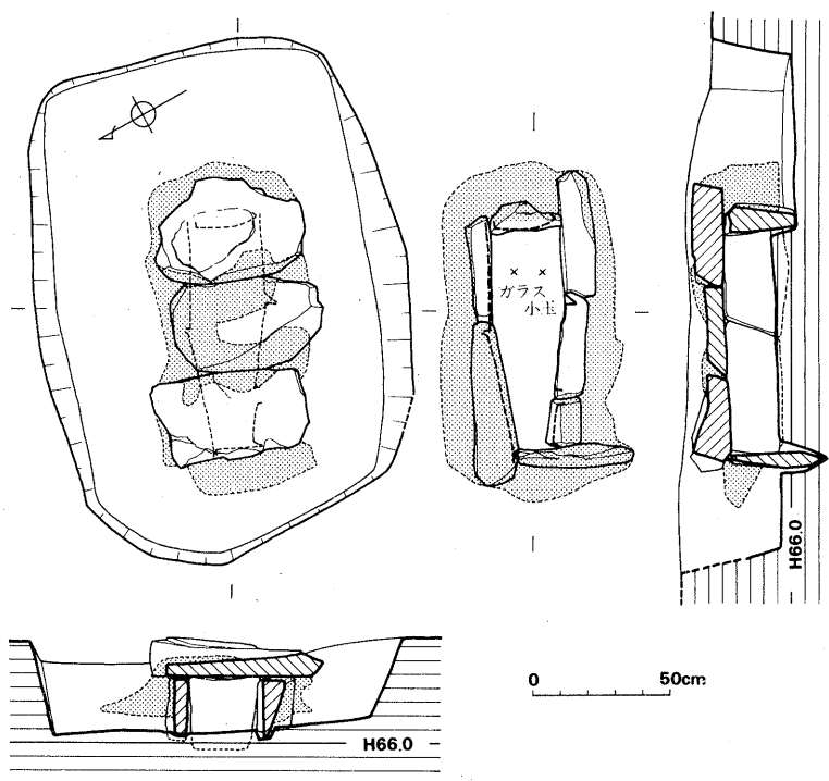
Fig. 6 1号墳第2主体 (1/30)
