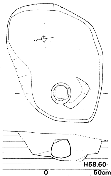
Fig. 38 4号墓 (1/20) 〈山本図〉
