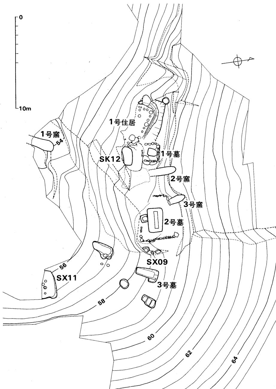
Fig.22 窯跡・墳墓群周辺地形図 (1/250)
