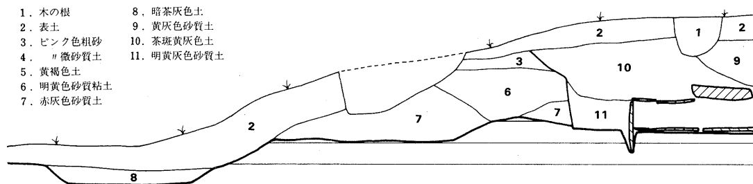
Fig. 7 1号墳土層図 (1/50)
