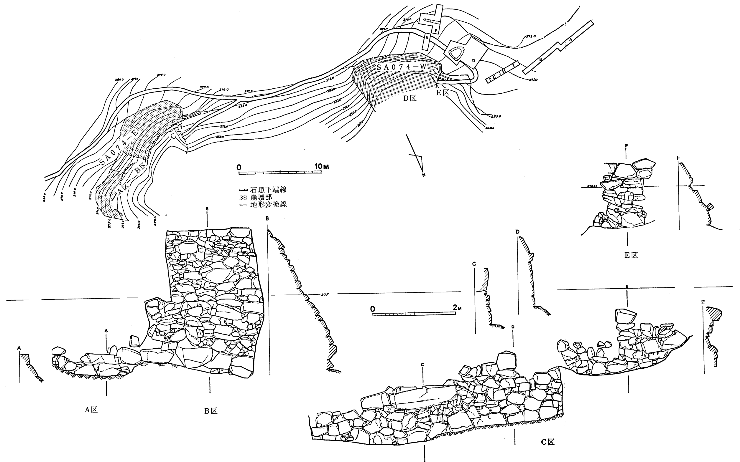
第7図 北石垣SA074地形図・石垣実測図
