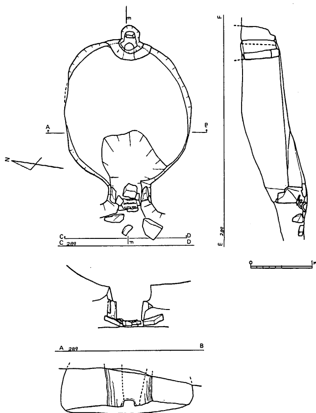
第5図 炭窯跡 SX072 実測図
