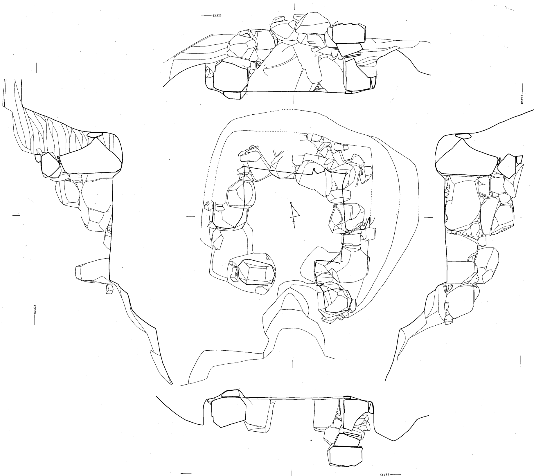
第27図 石室実測図 (1/40)
