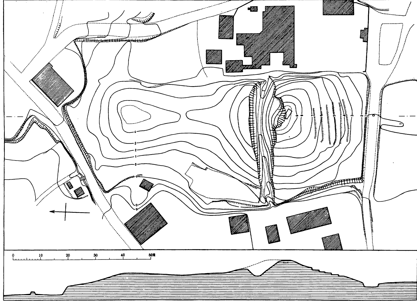
圖 版 第 二 遺 蹟 外 形 Pl. II. Plan and Section of the Mound
