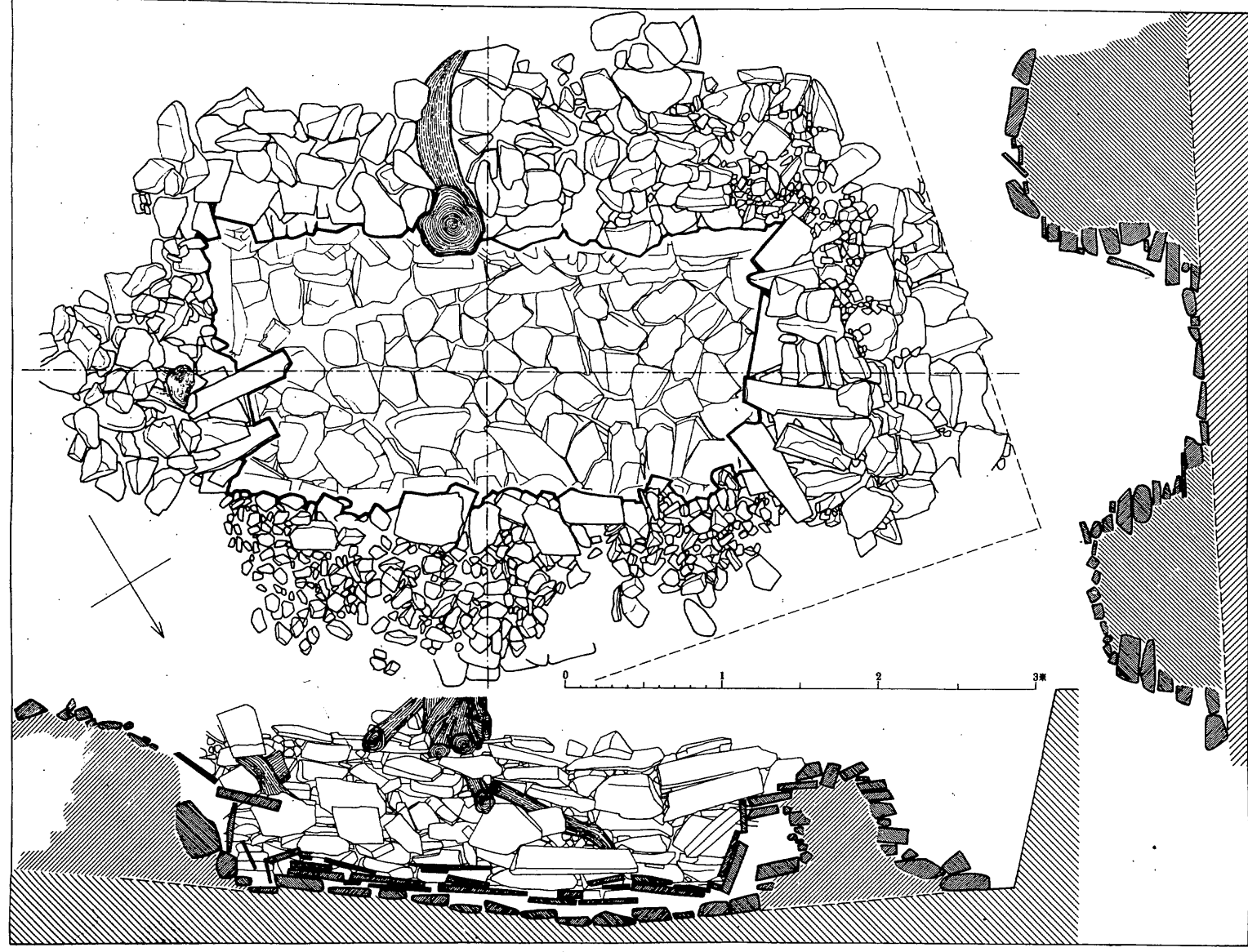
鏡子塚古墳竪穴式石室實測圖
