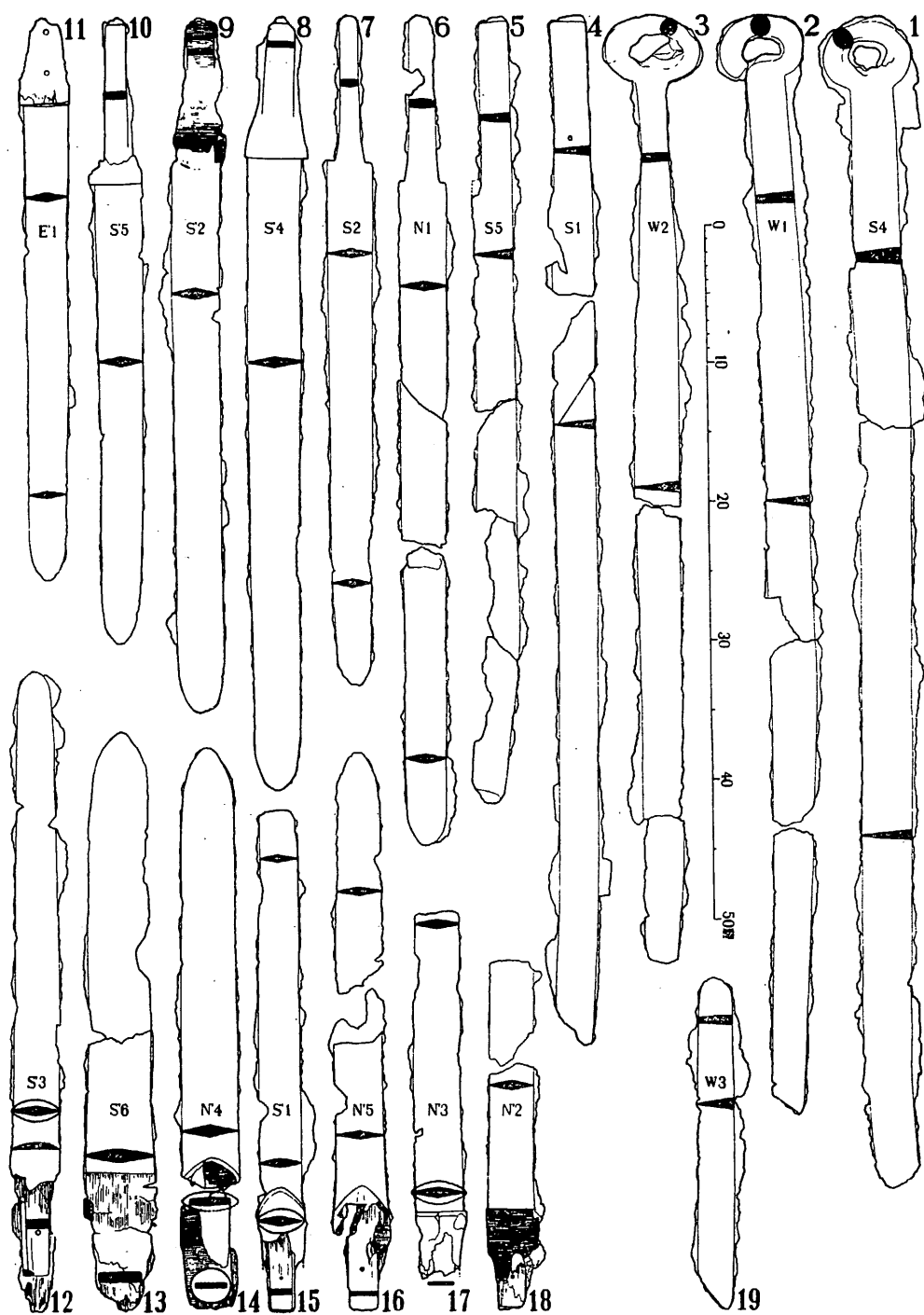
第十一圖 銚子塚古墳發見刀劍類實測圖 Fig. 11.
