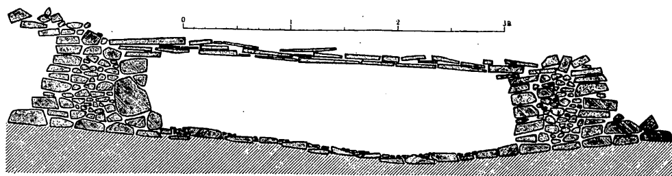
第五圖 石室天井部構造復原圖 Fig. 5.
