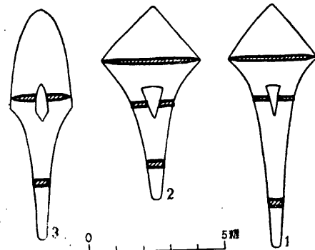
第十二圖 銚子塚古墳發見鐵鏃實測圖 Fig. 12.
